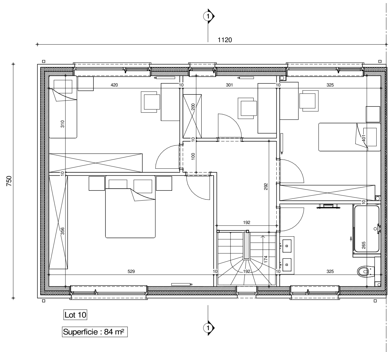
ETAGE
