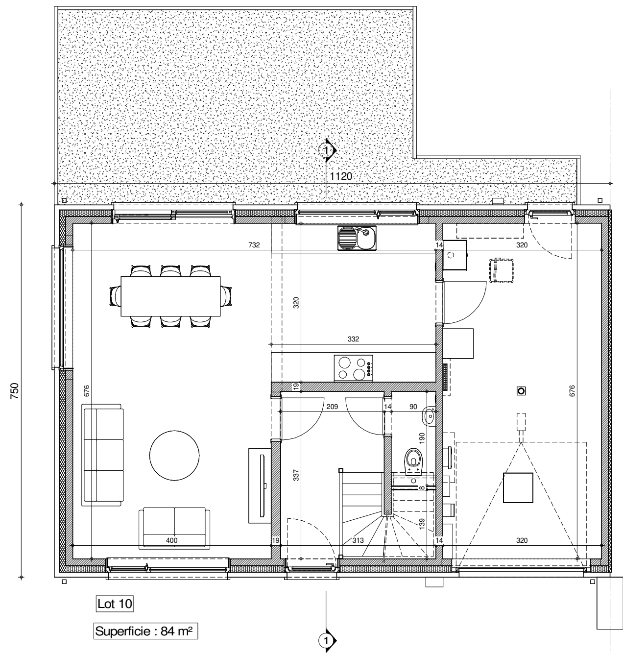
REZ-DE-CHAUSSEE
