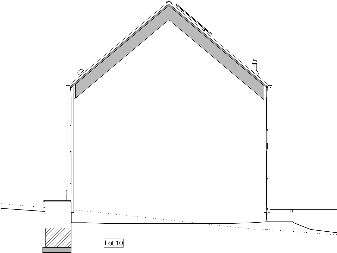
PIGNON DROIT
