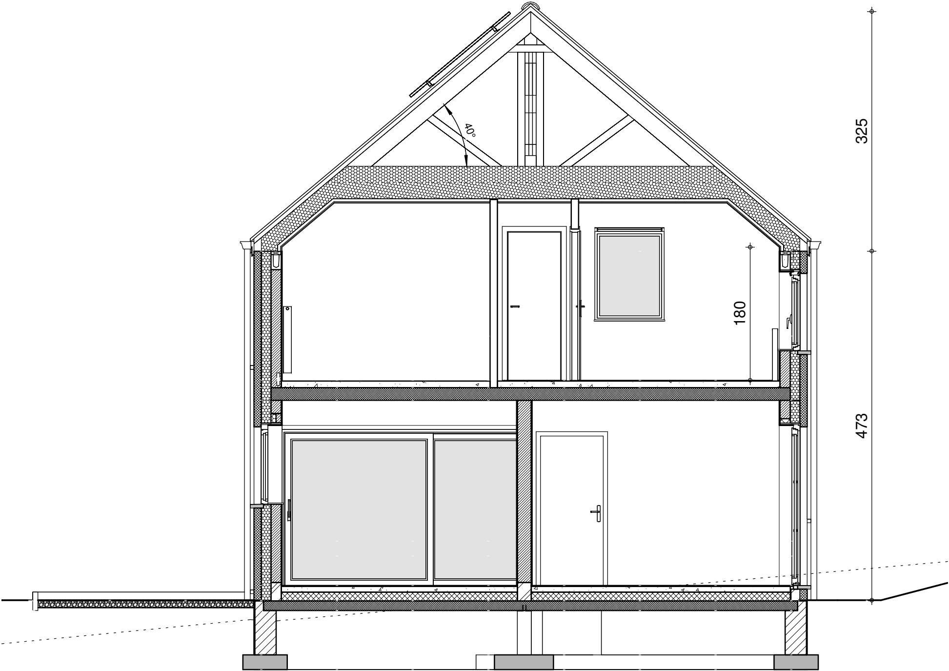
COUPE A-A
