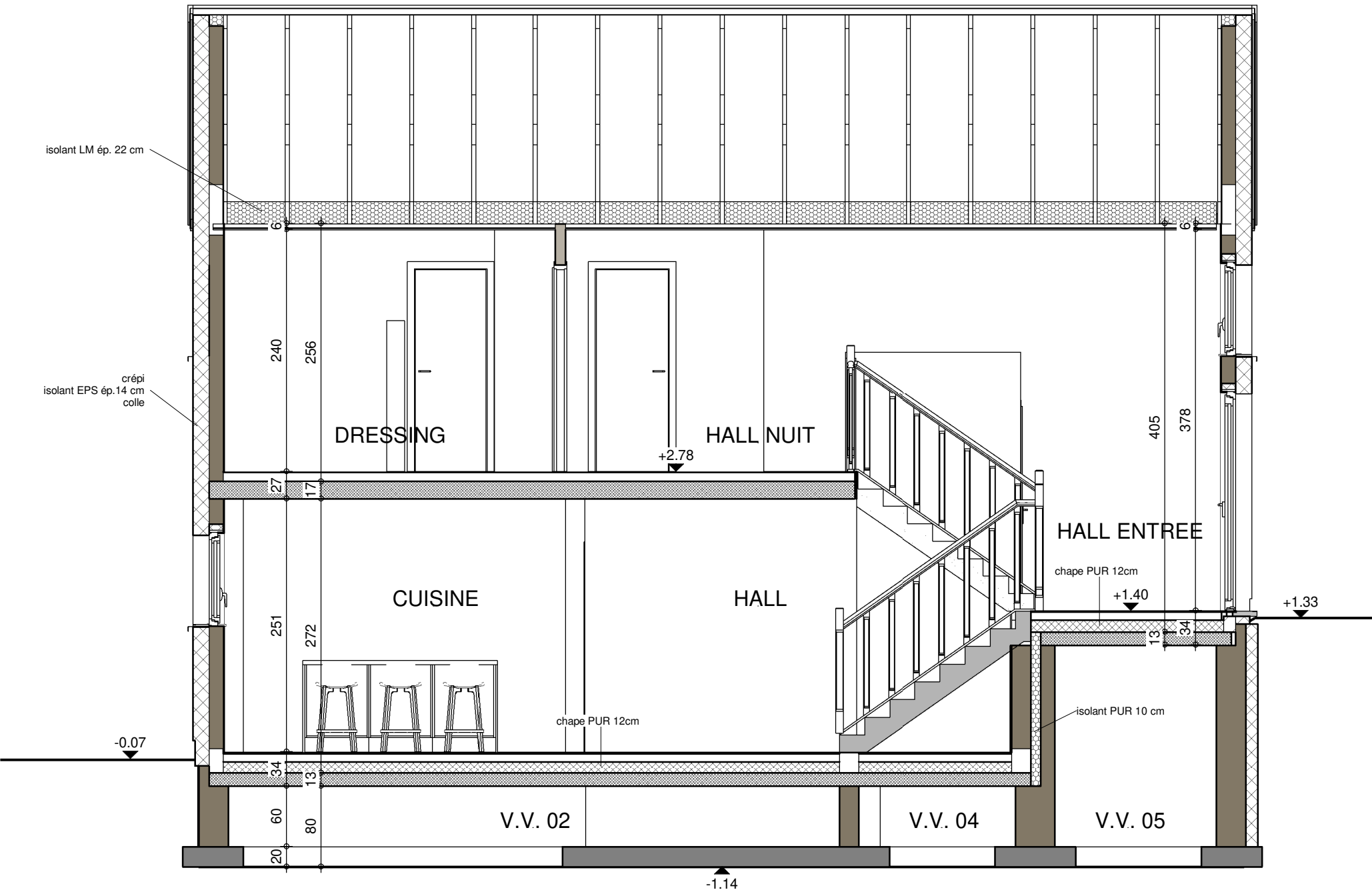
COUPE BB
