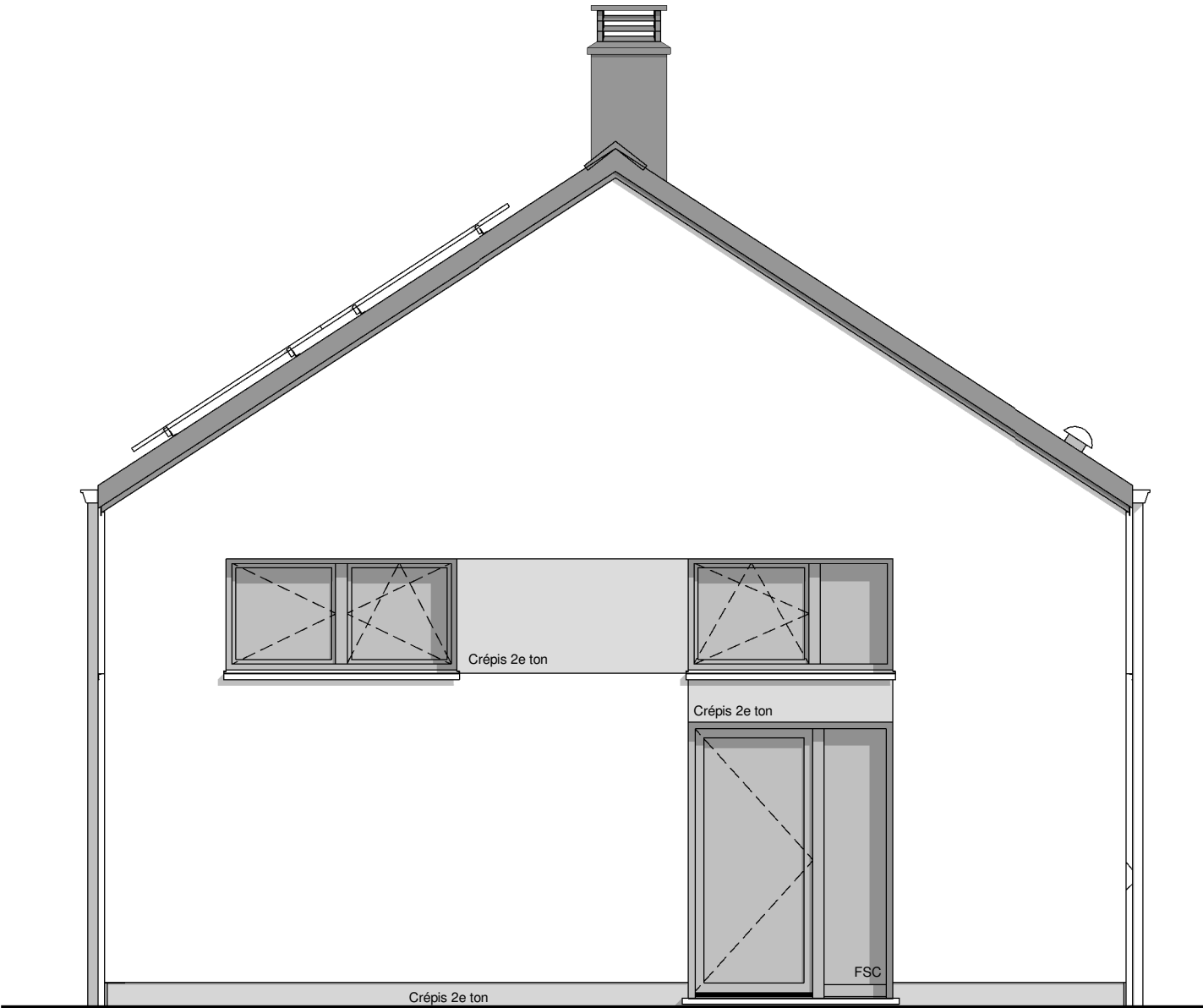
PIGNON AVANT
