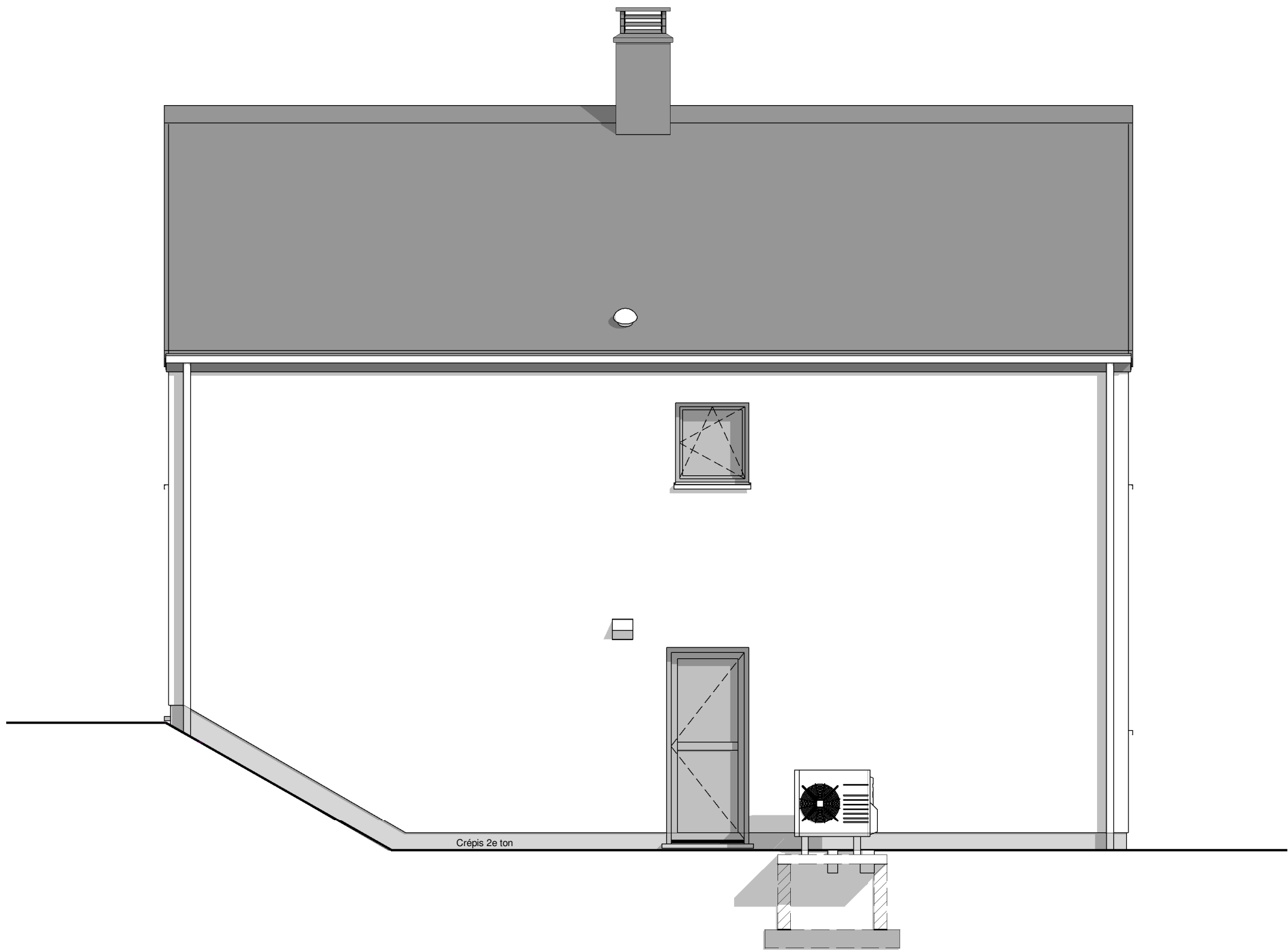
FACADE DROITE
