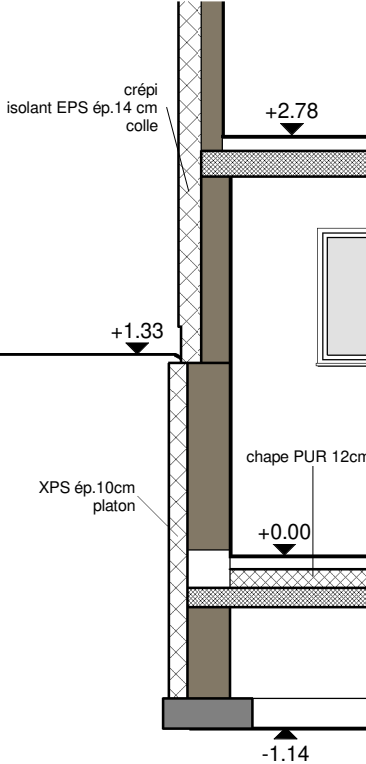
COUPE CC
