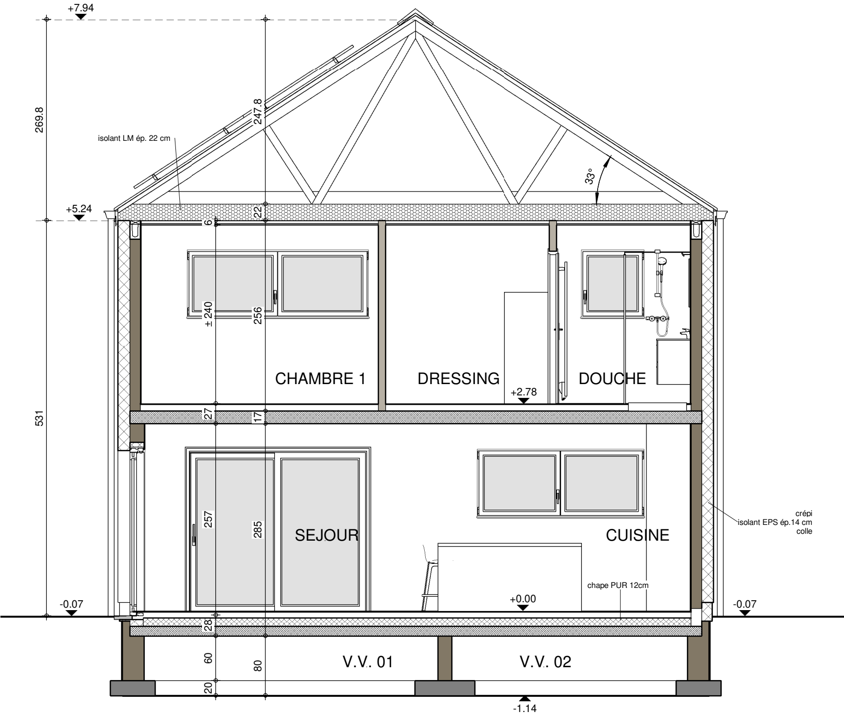
COUPE AA
