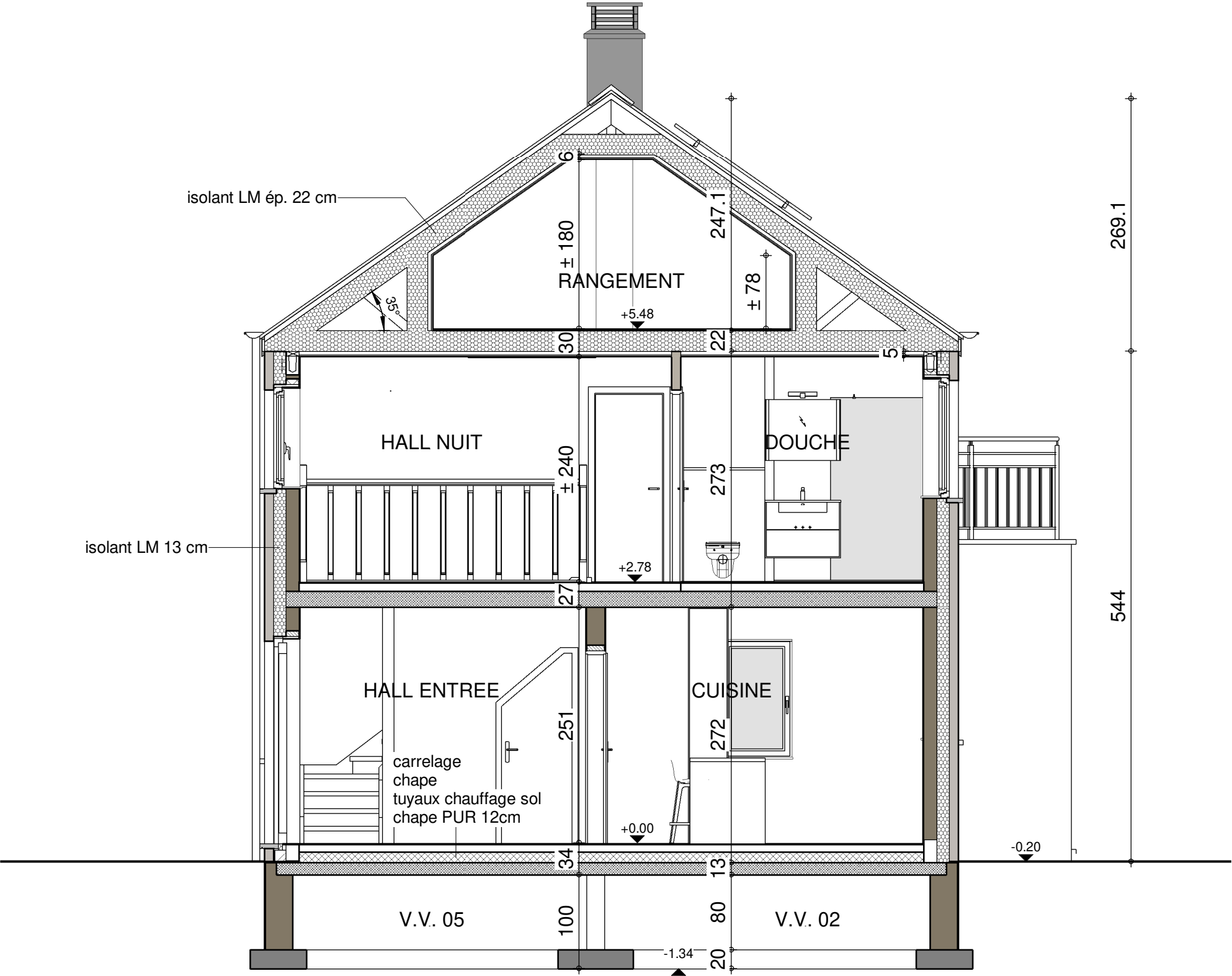
COUPE AA
