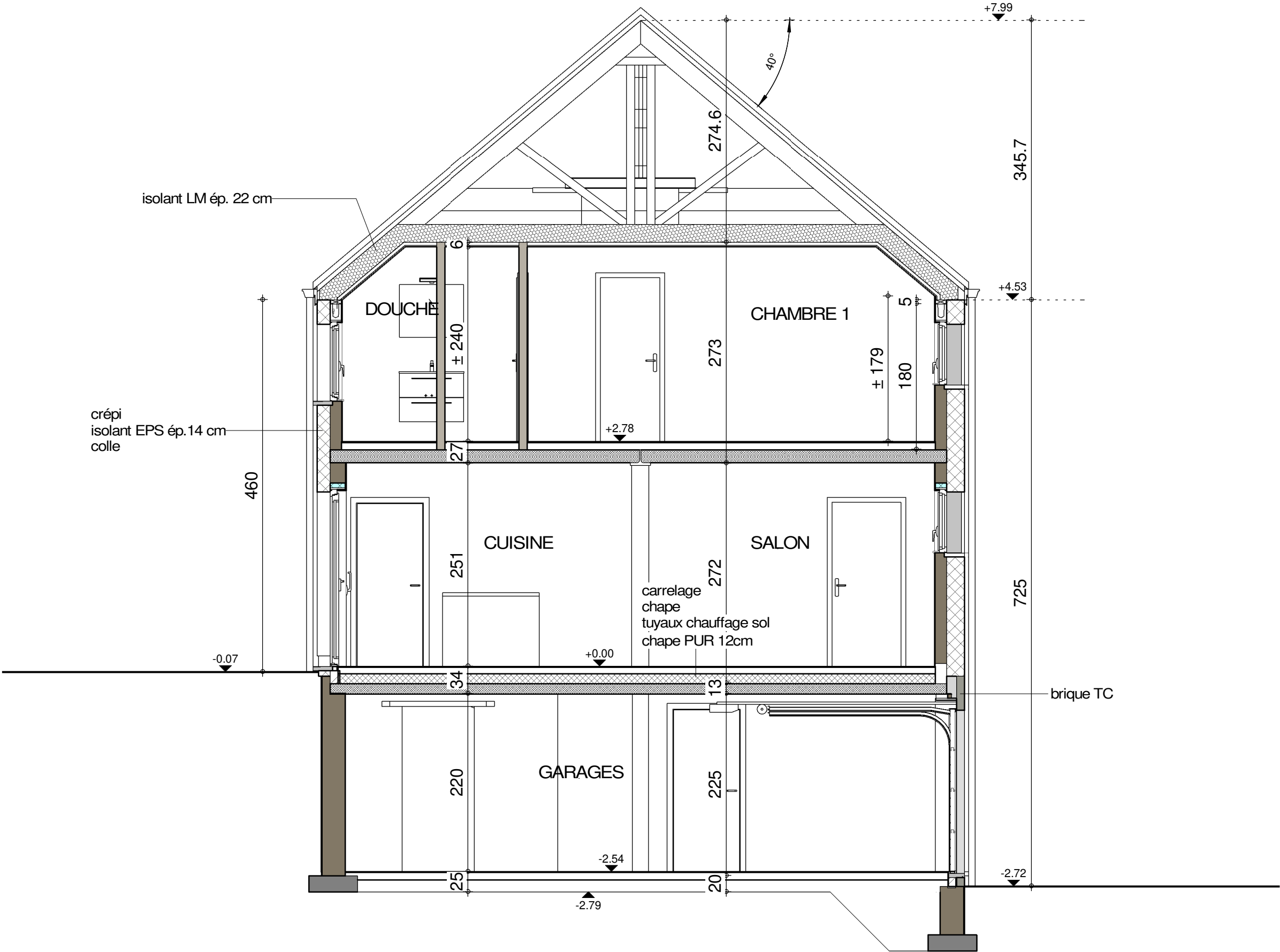
COUPE AA
