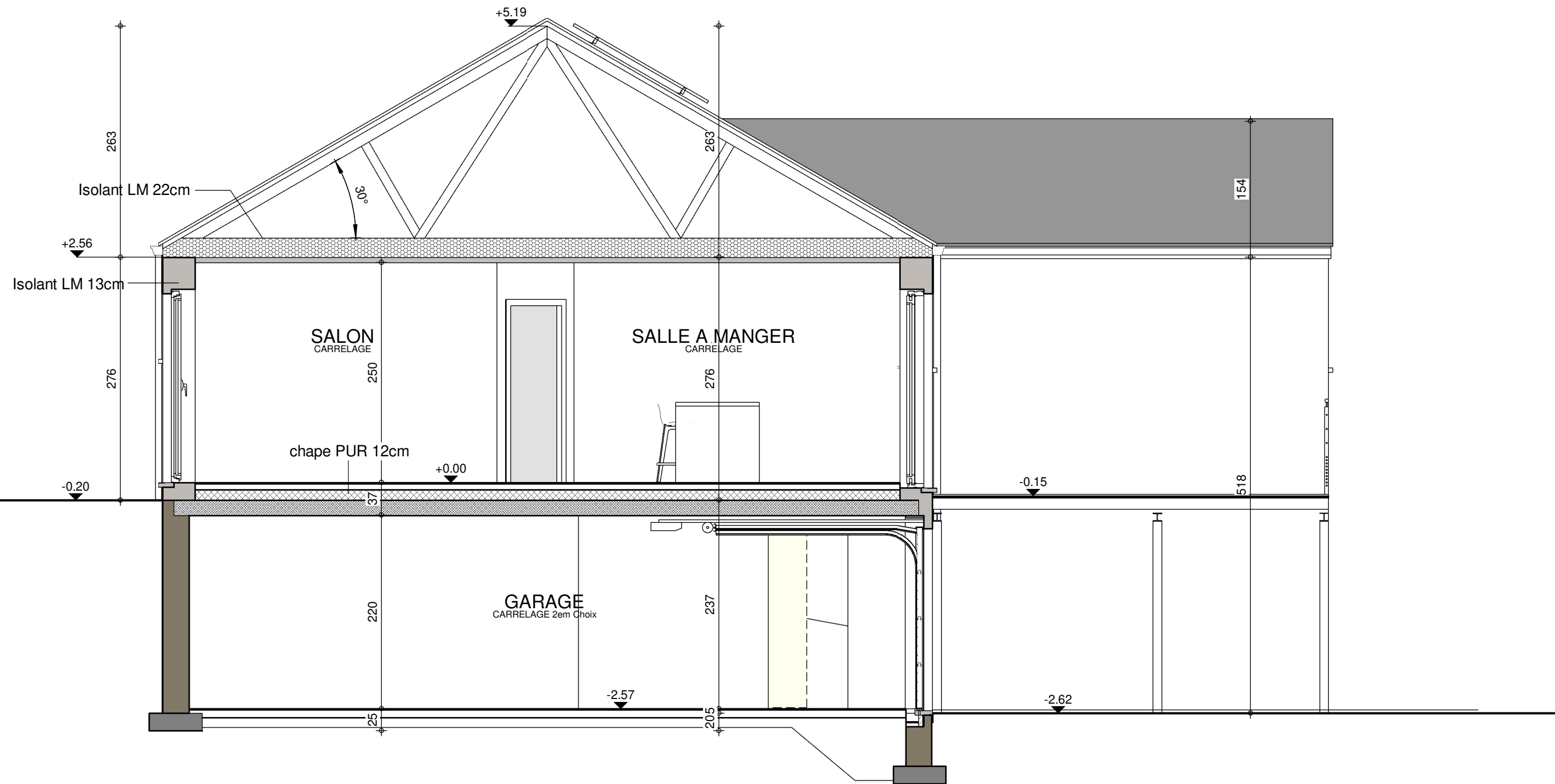
COUPE AA
