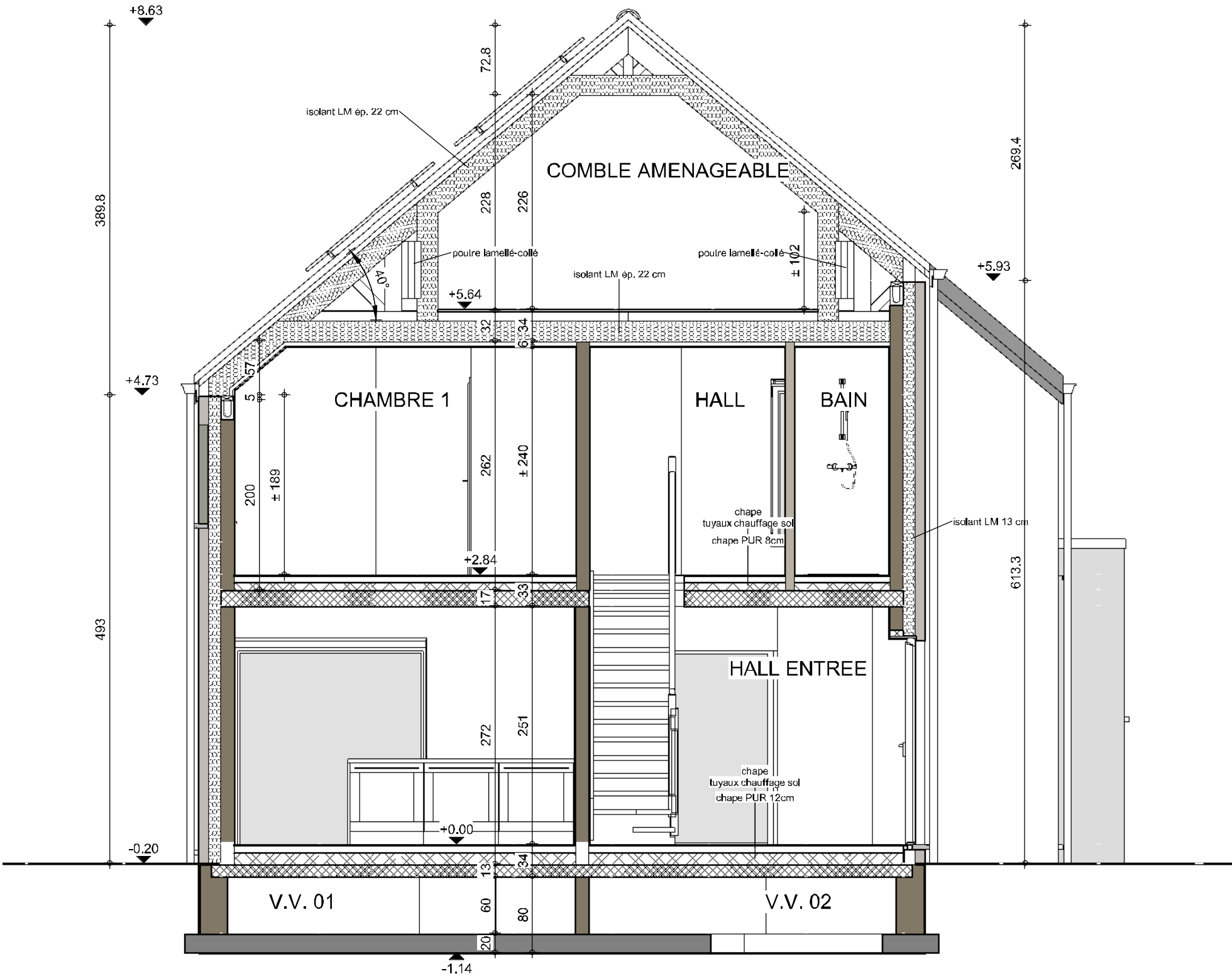
COUPE AA
