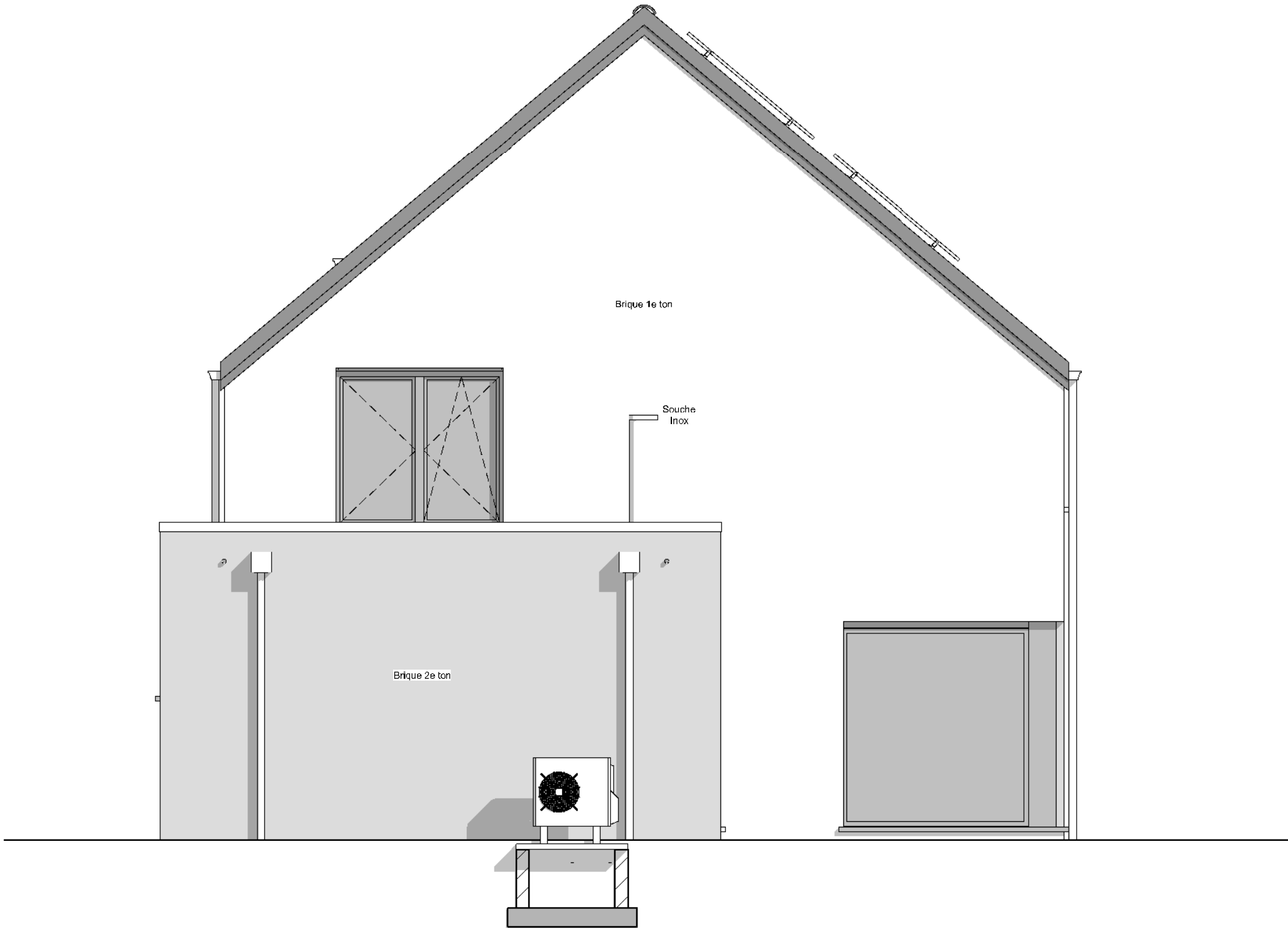
PIGNON DROIT
