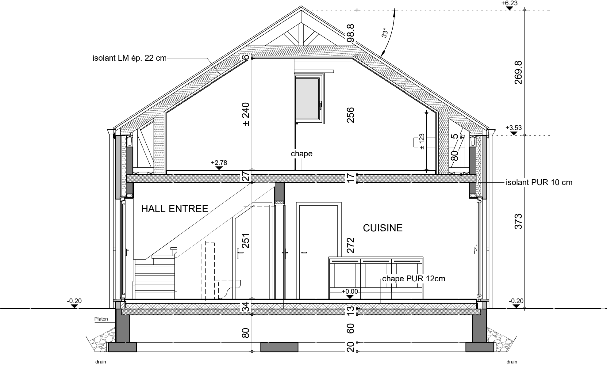
COUPE AA
