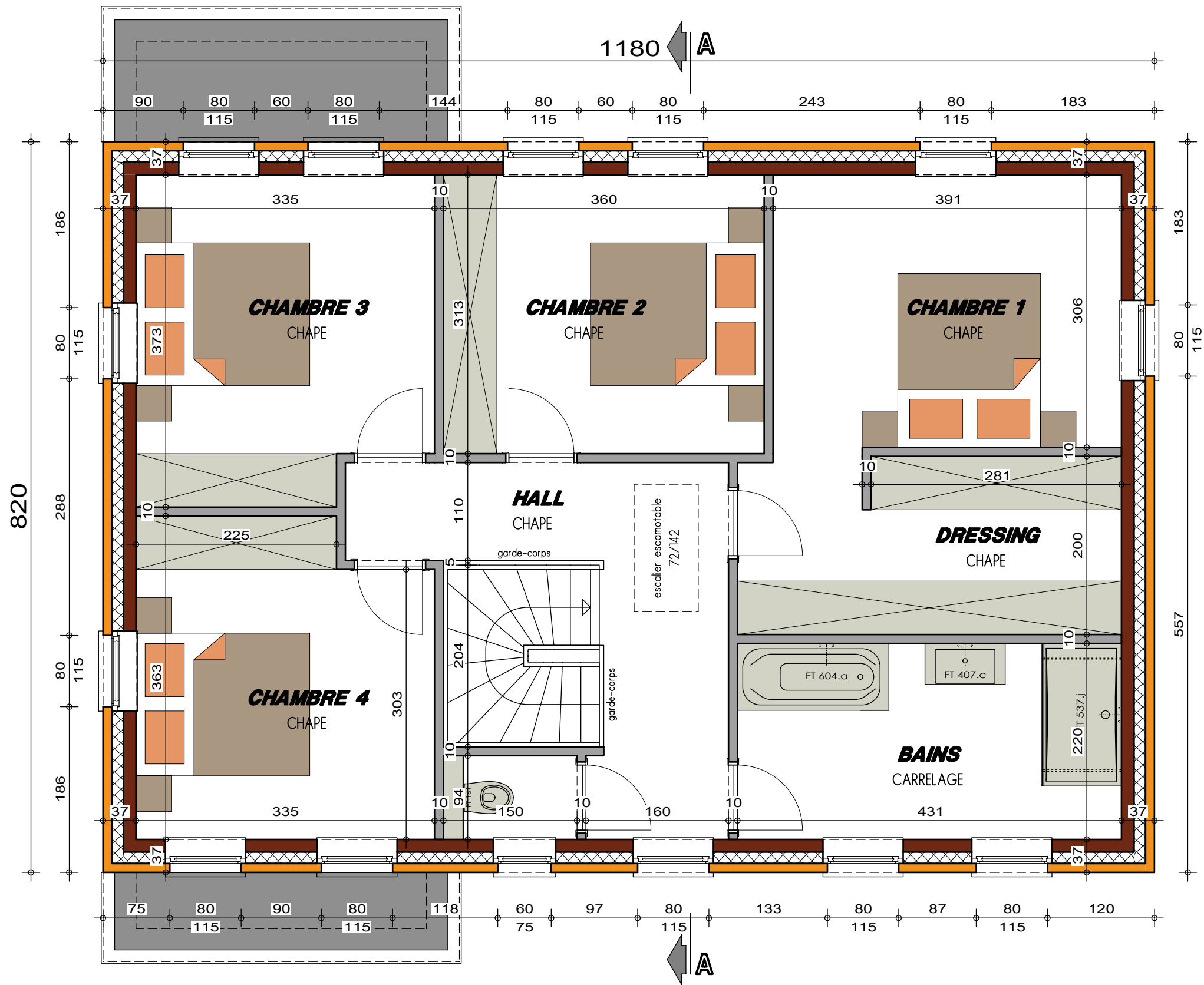
PLAN ETAGE
