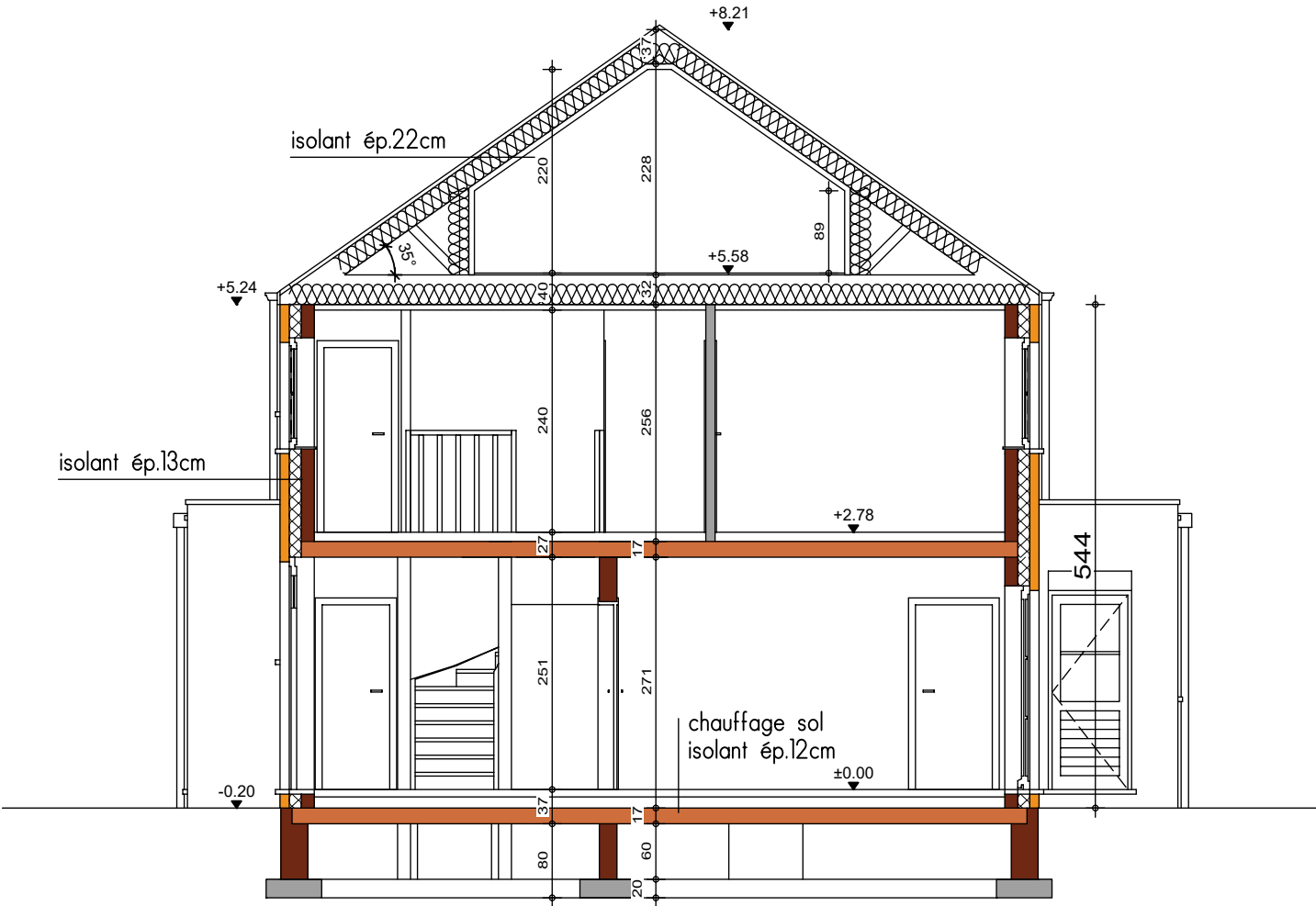
COUPE AA
