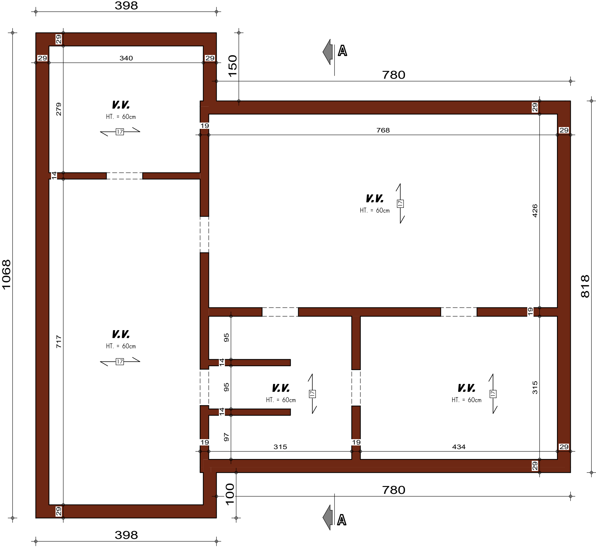
PLAN SOUS-SOL
