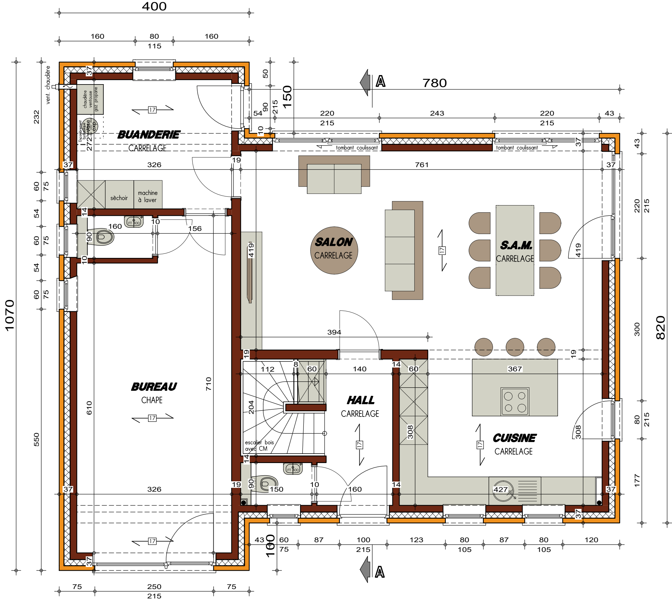
PLAN REZ-DE-CHAUSSEE
