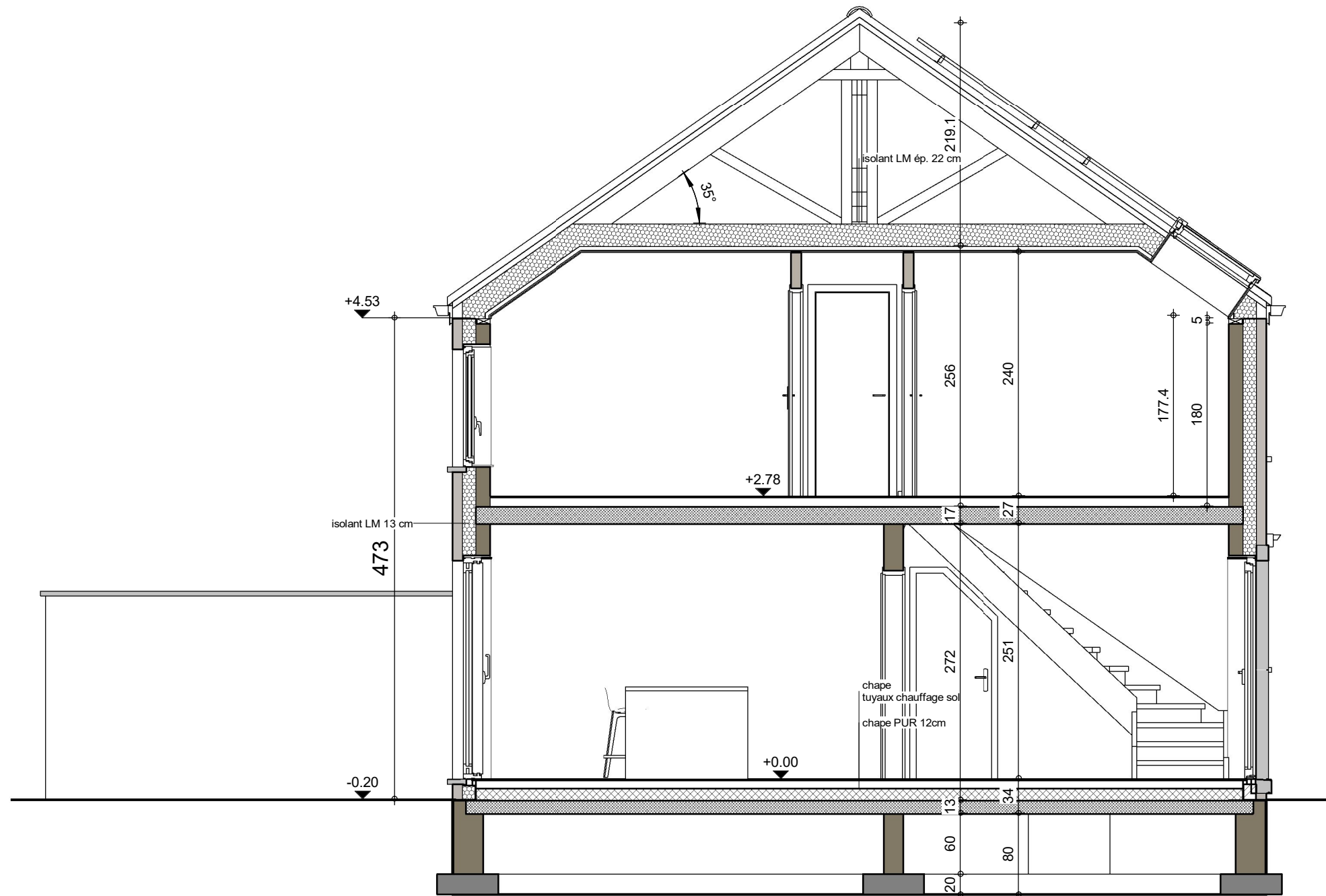
COUPE AA
