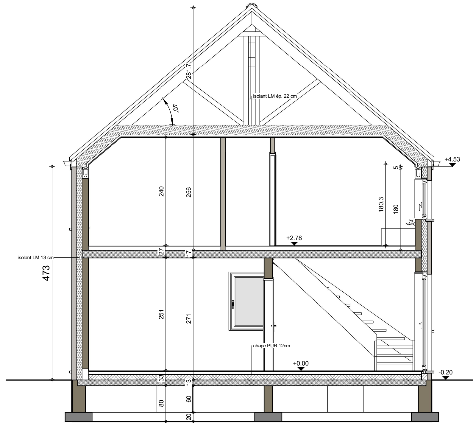
COUPE AA
