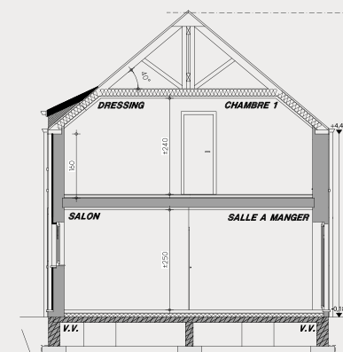
Coupe AA
