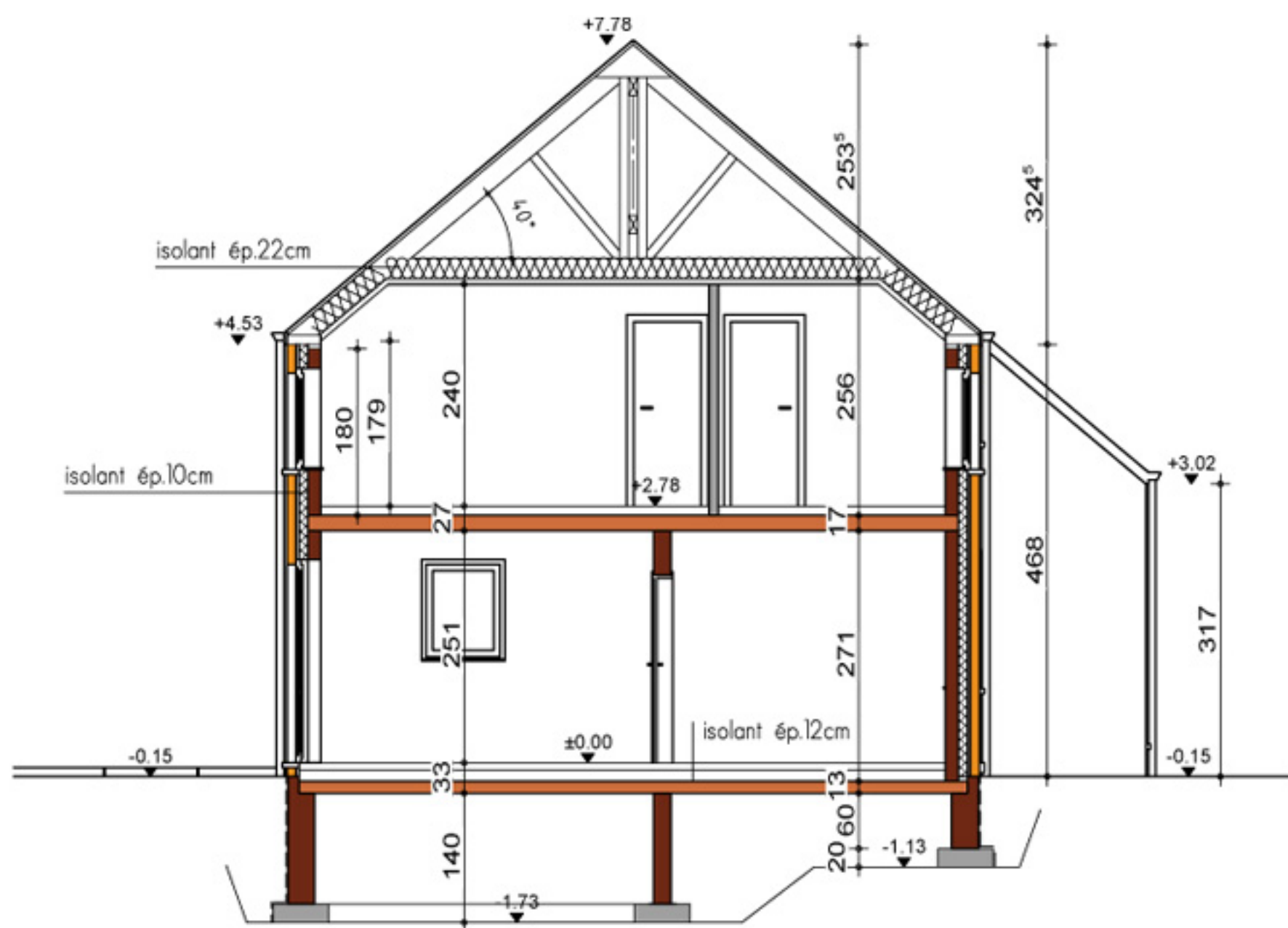
COUPE AA
