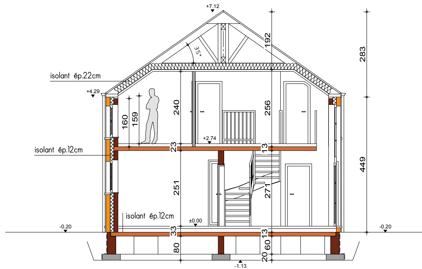
COUPE AA
