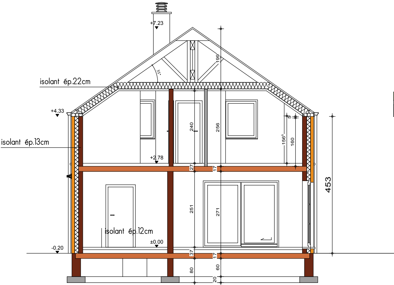
COUPE AA
