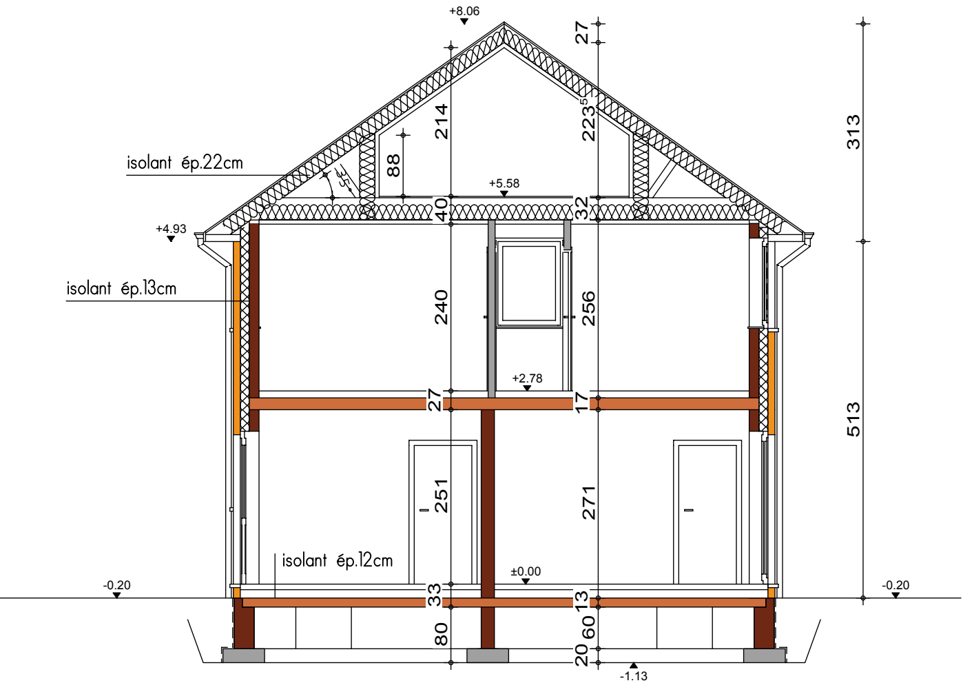
COUPE AA
