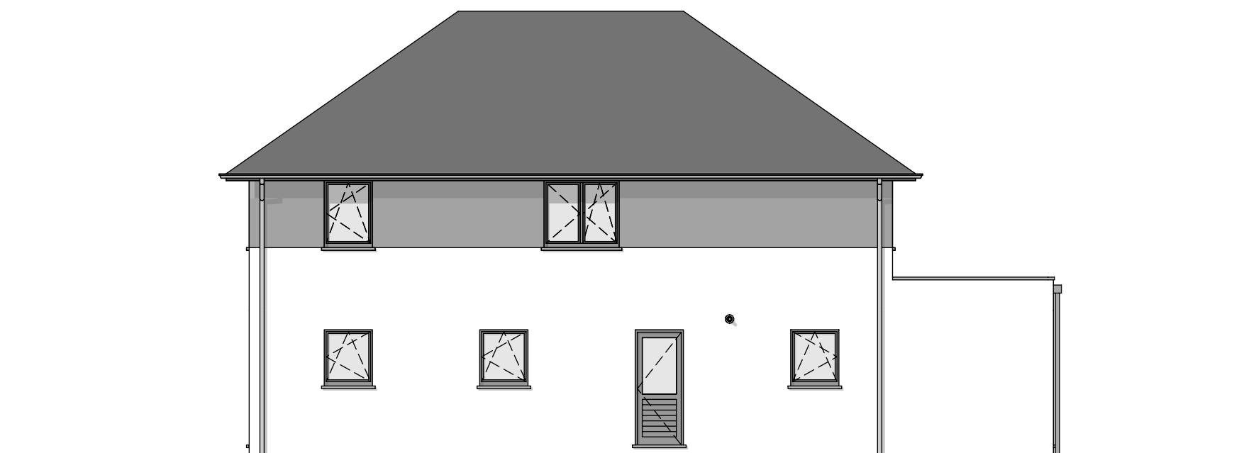
FACADE LATERALE DROITE
