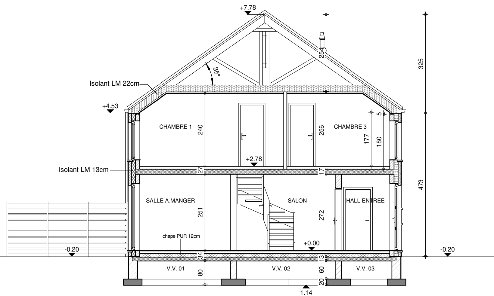
COUPE AA
