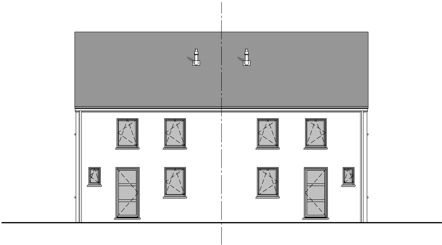
FACADE AVANT
