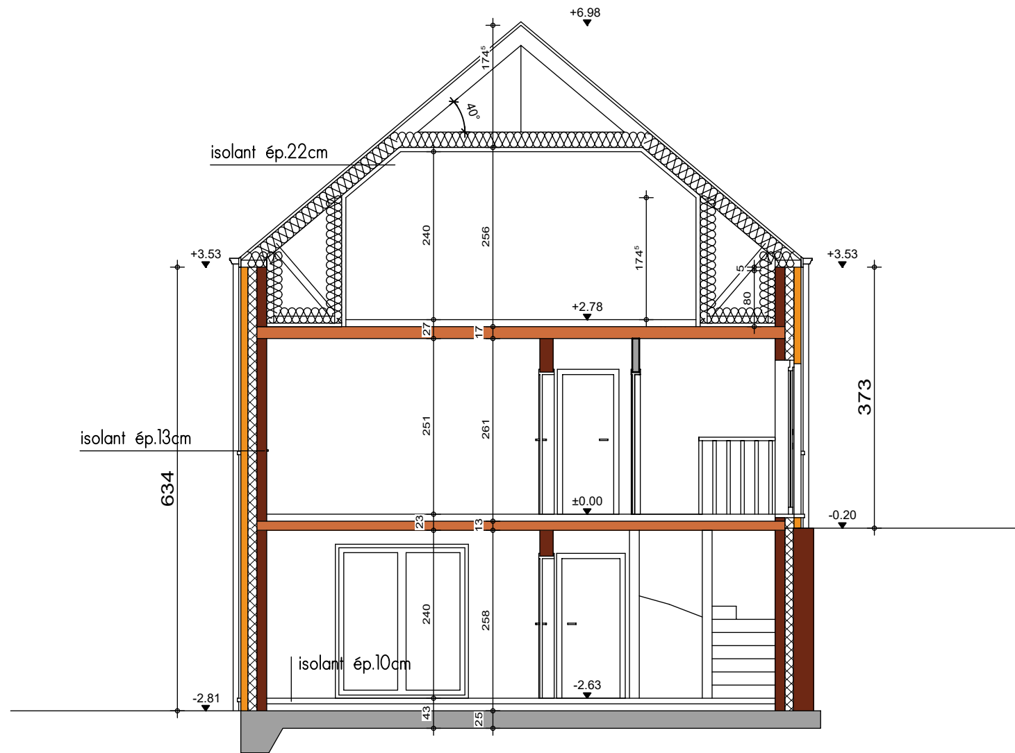
COUPE AA
