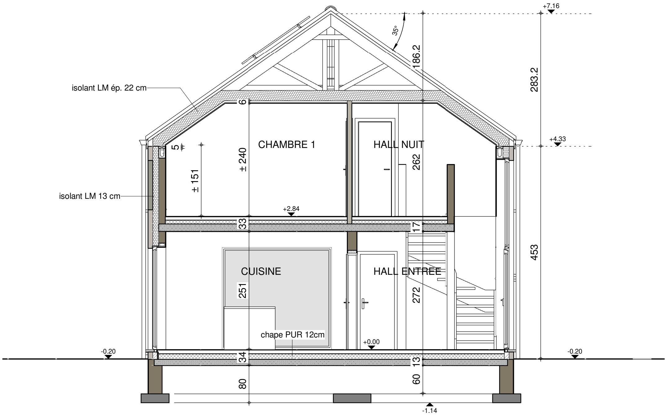
COUPE AA
