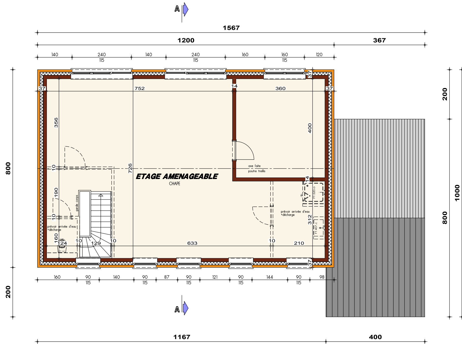
PLAN ETAGE
