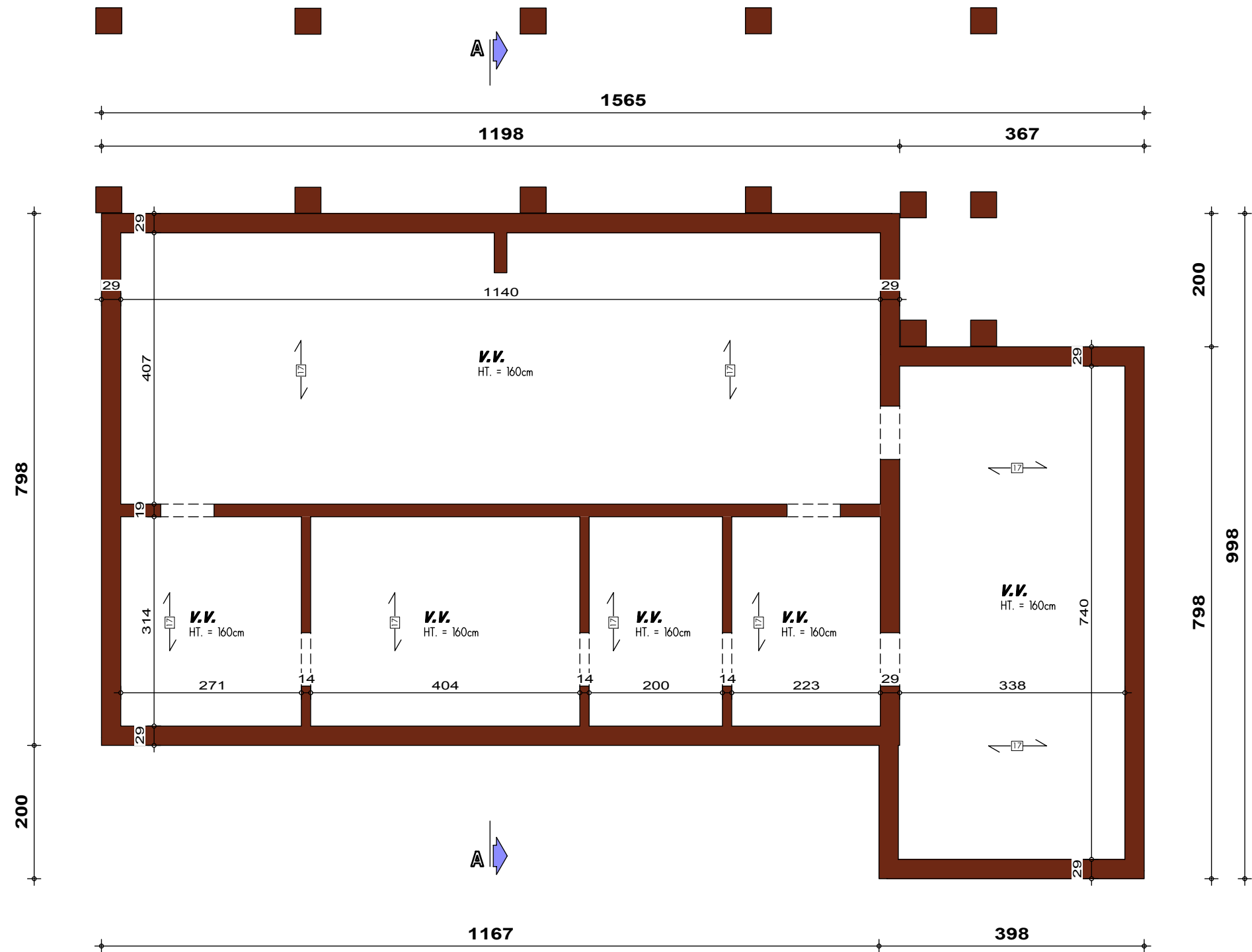
PLAN SOUS-SOL
