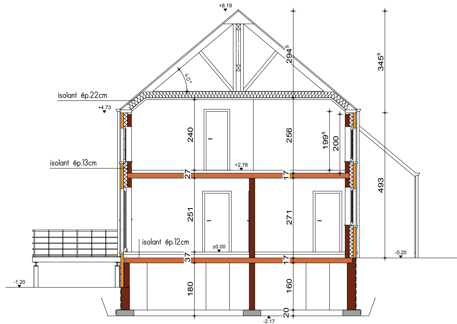
COUPE AA
