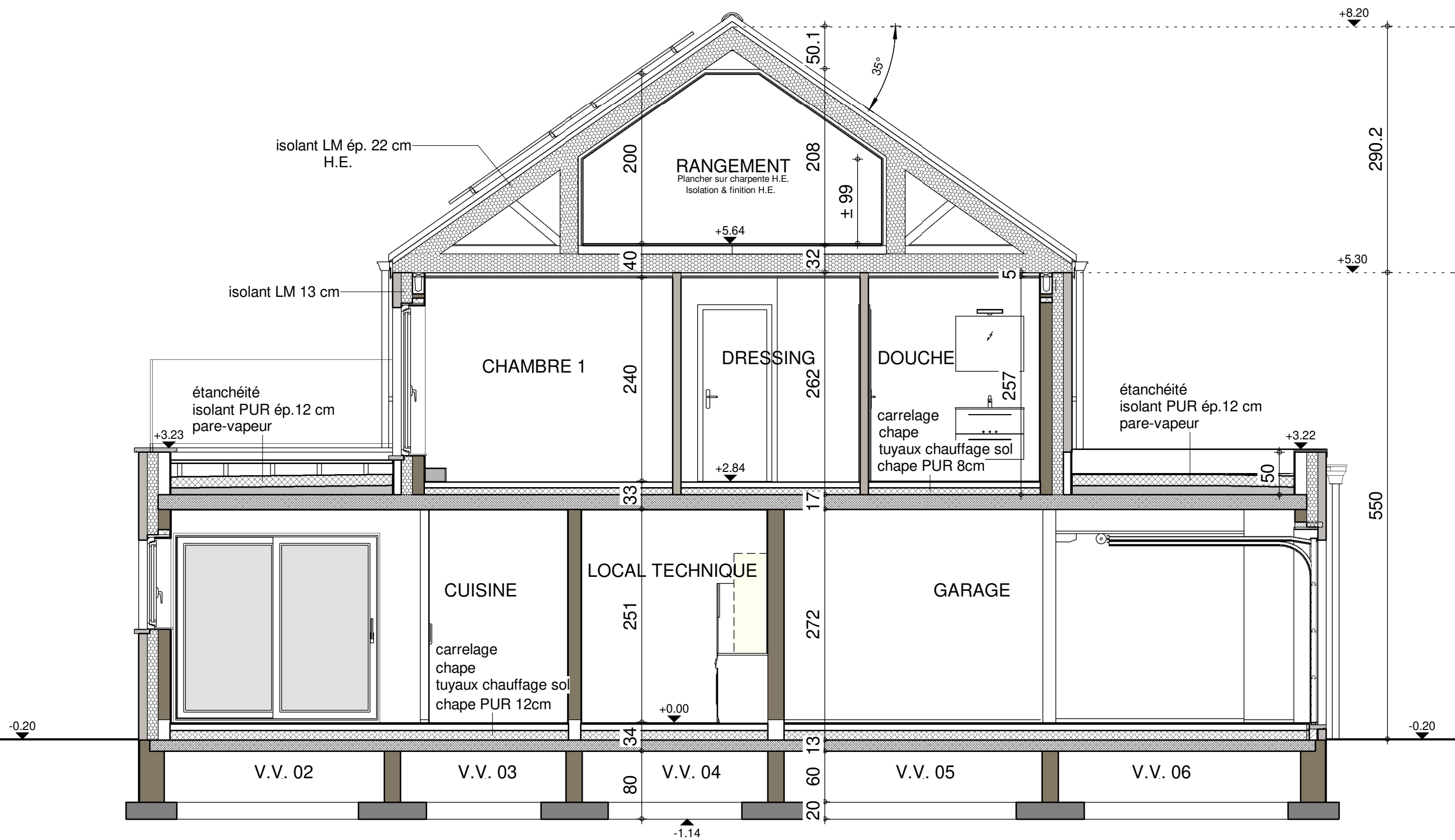
COUPE AA
