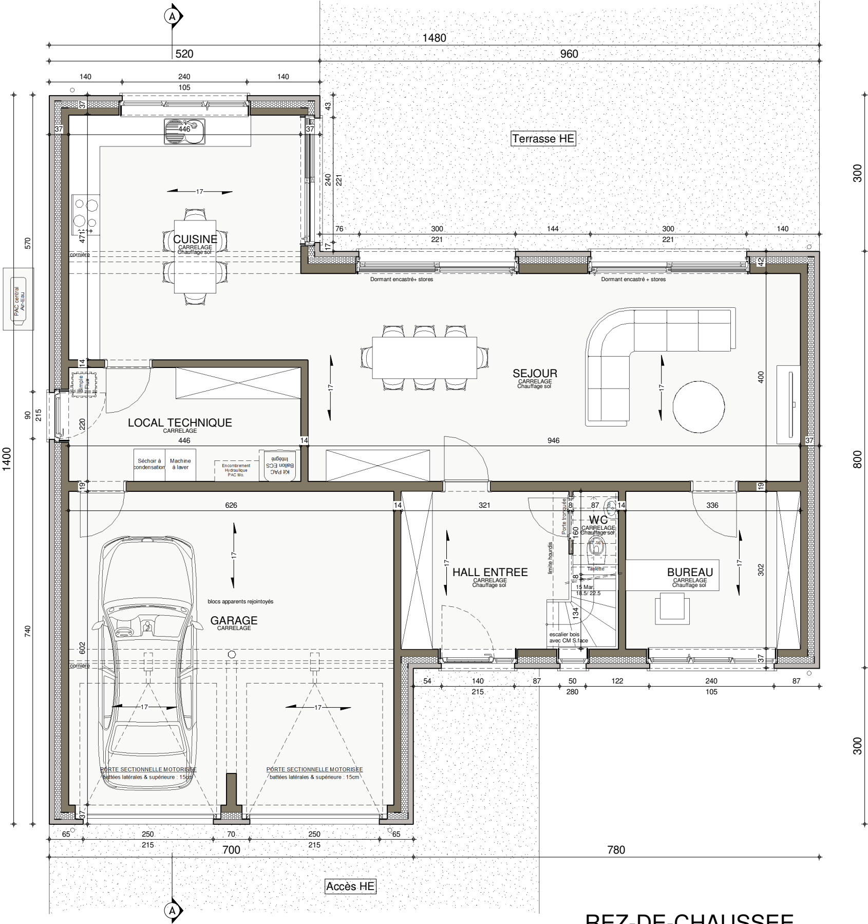
REZ-DE-CHAUSSEE
