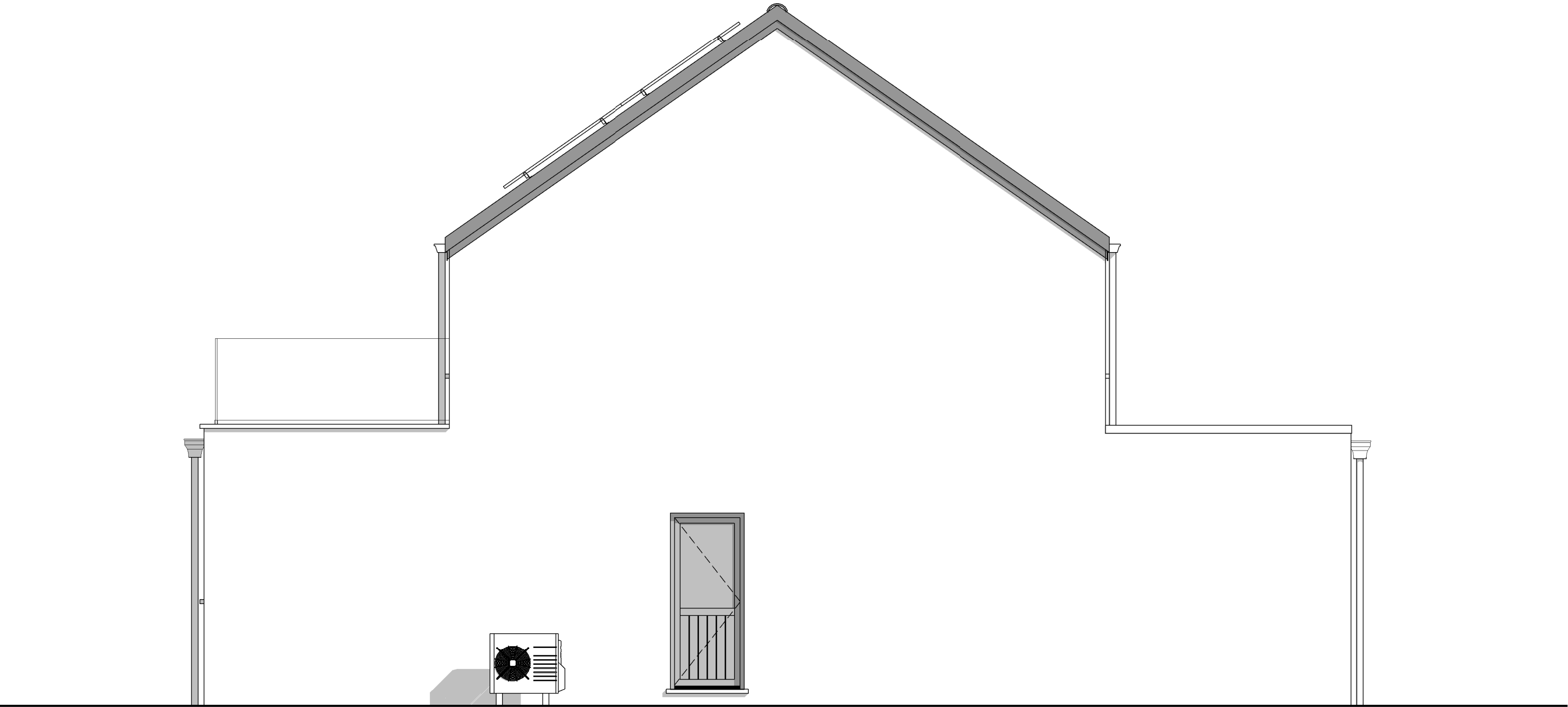
PIGNON GAUCHE
