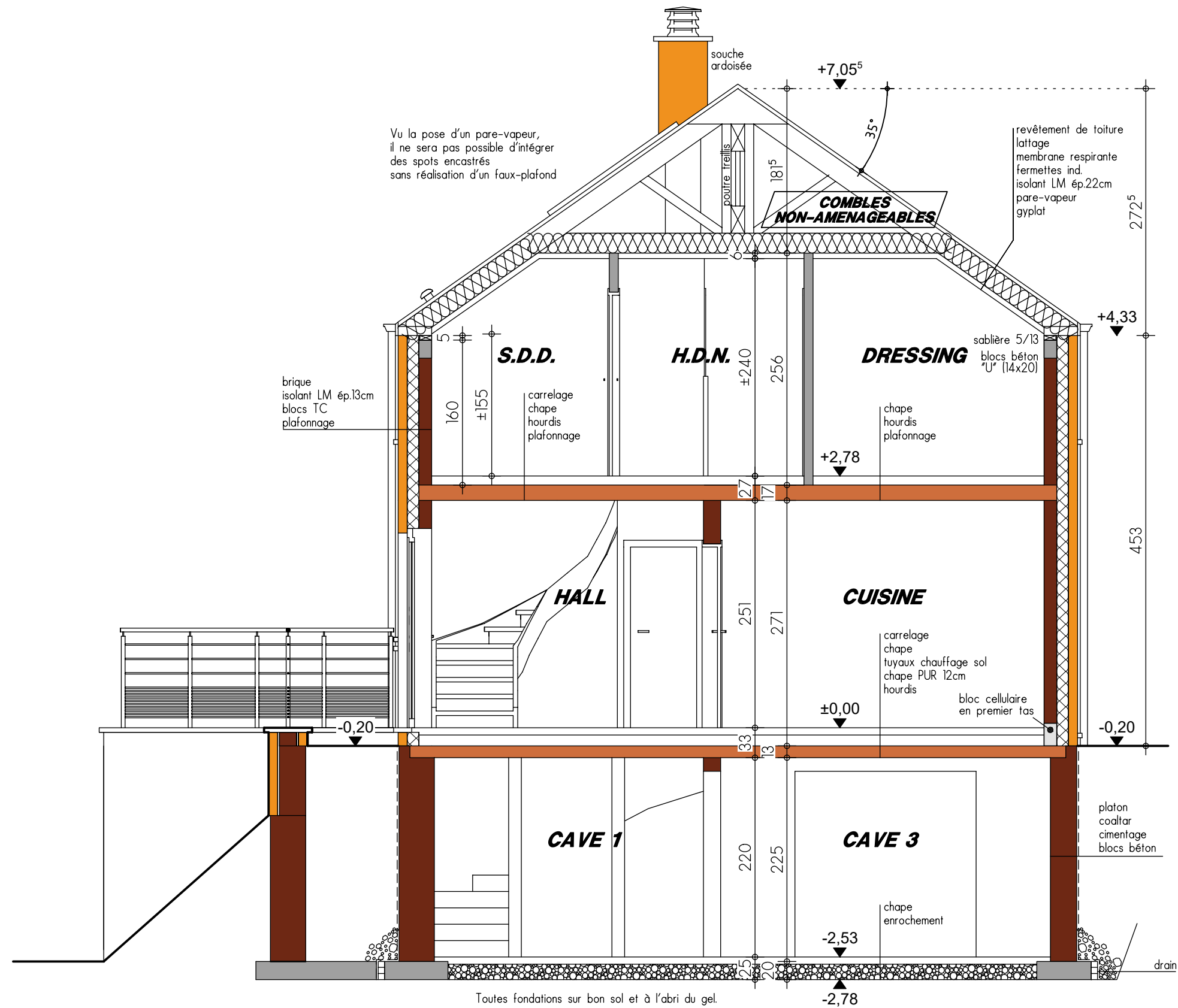
COUPE AA
