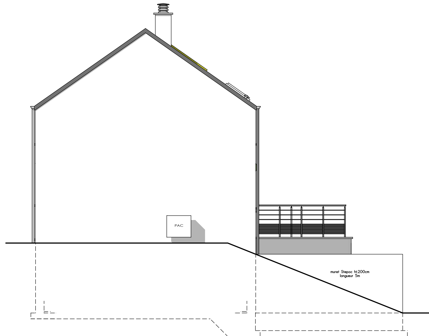
PIGNON GAUCHE
