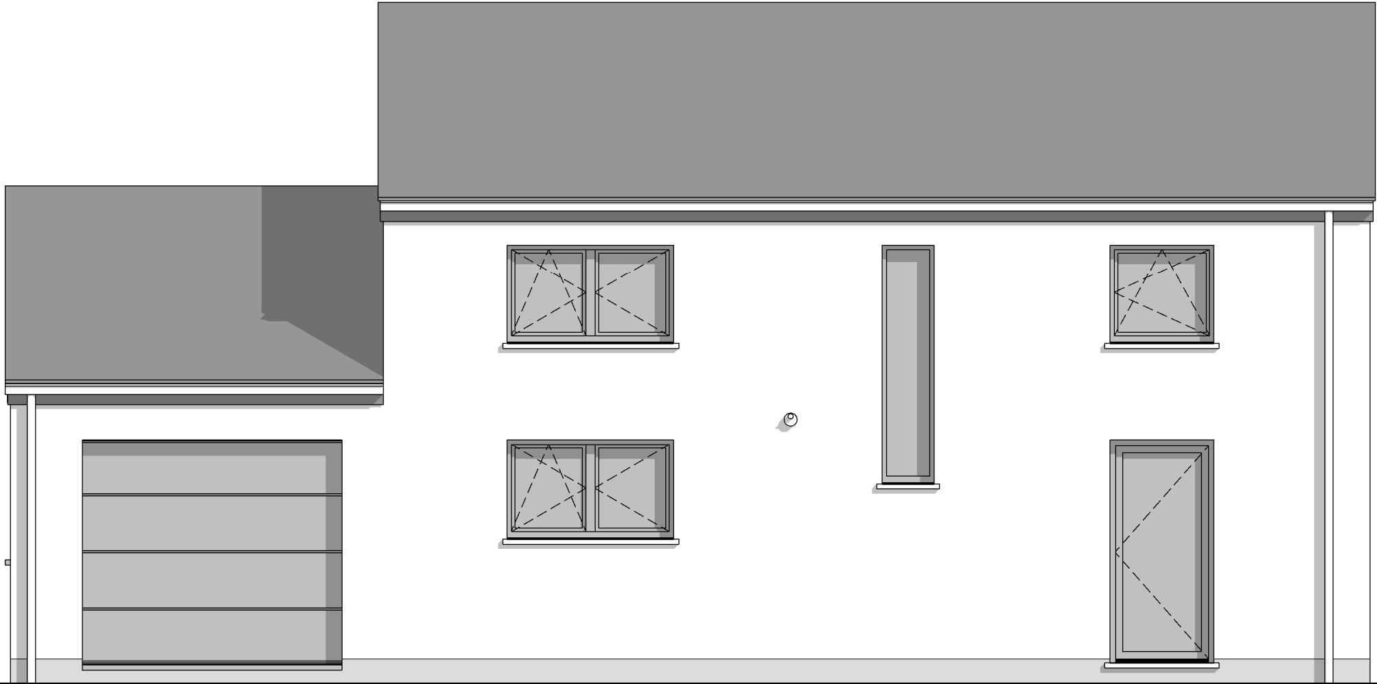
FACADE AVANT
