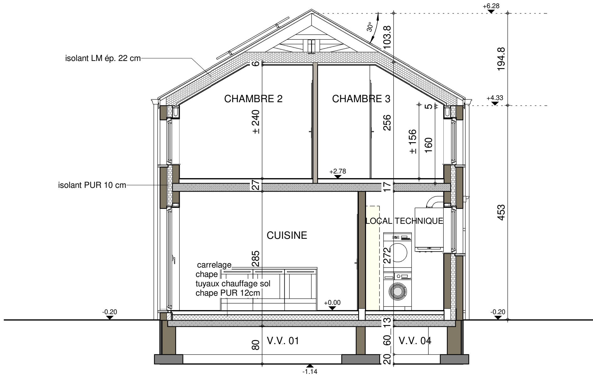
COUPE AA
