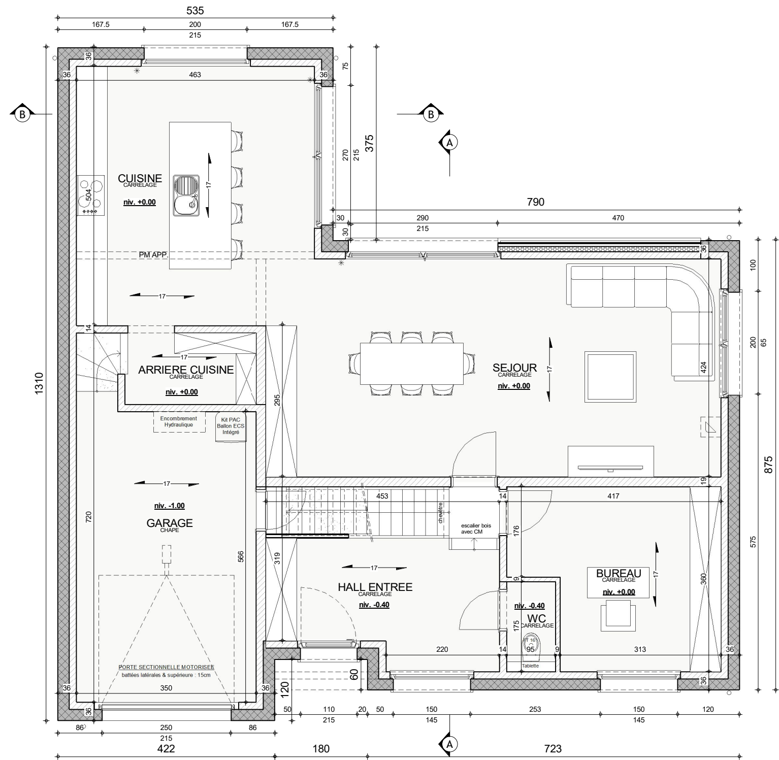
REZ-DE-CHAUSSEE
