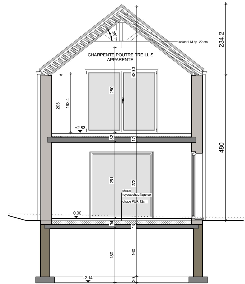
COUPE BB
