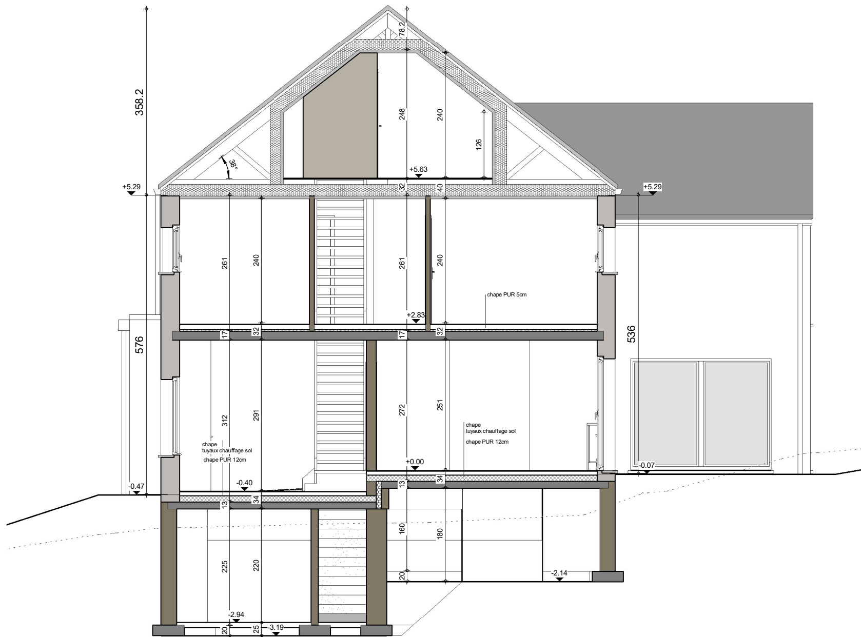
COUPE AA
