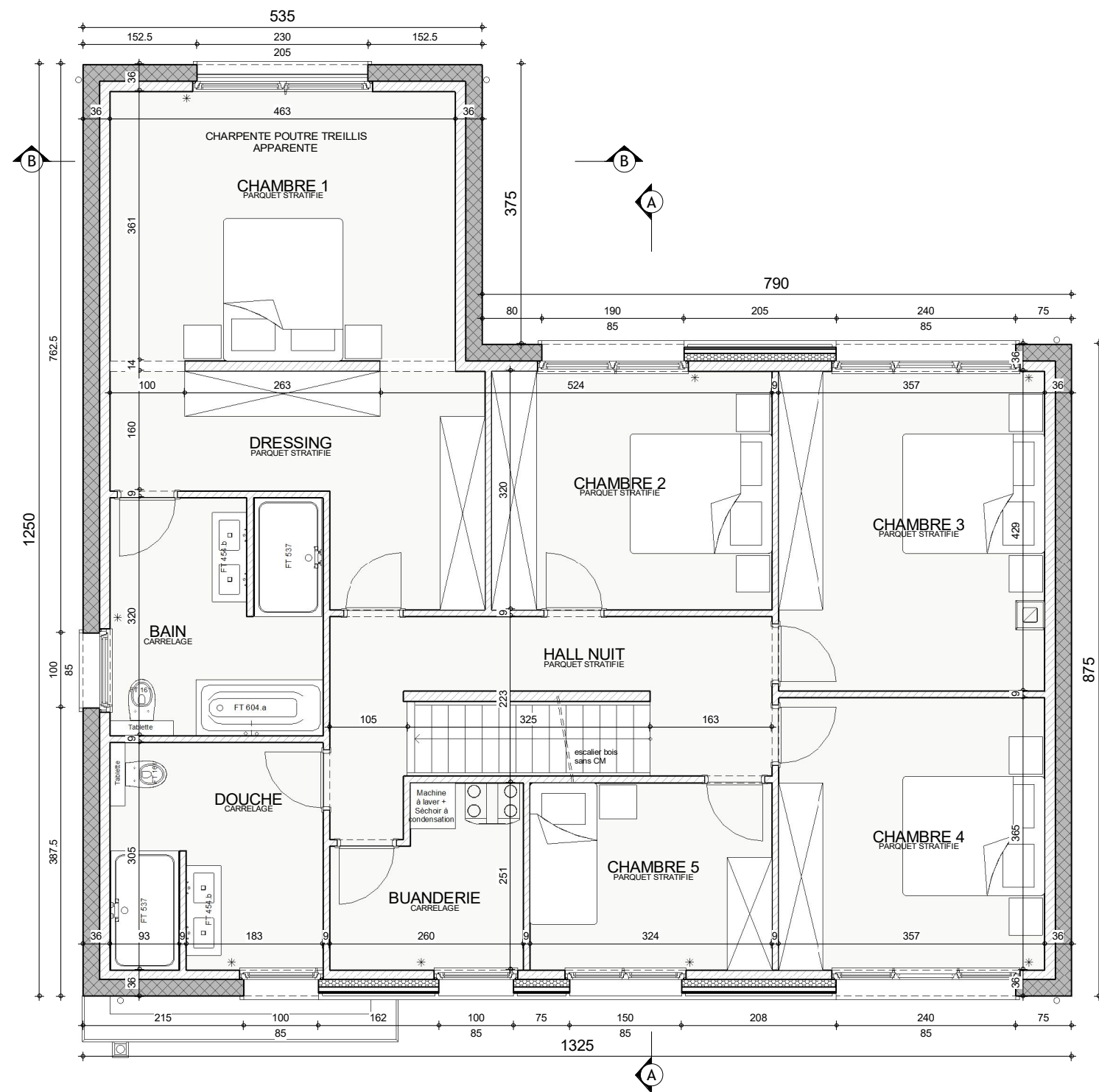
ETAGE
