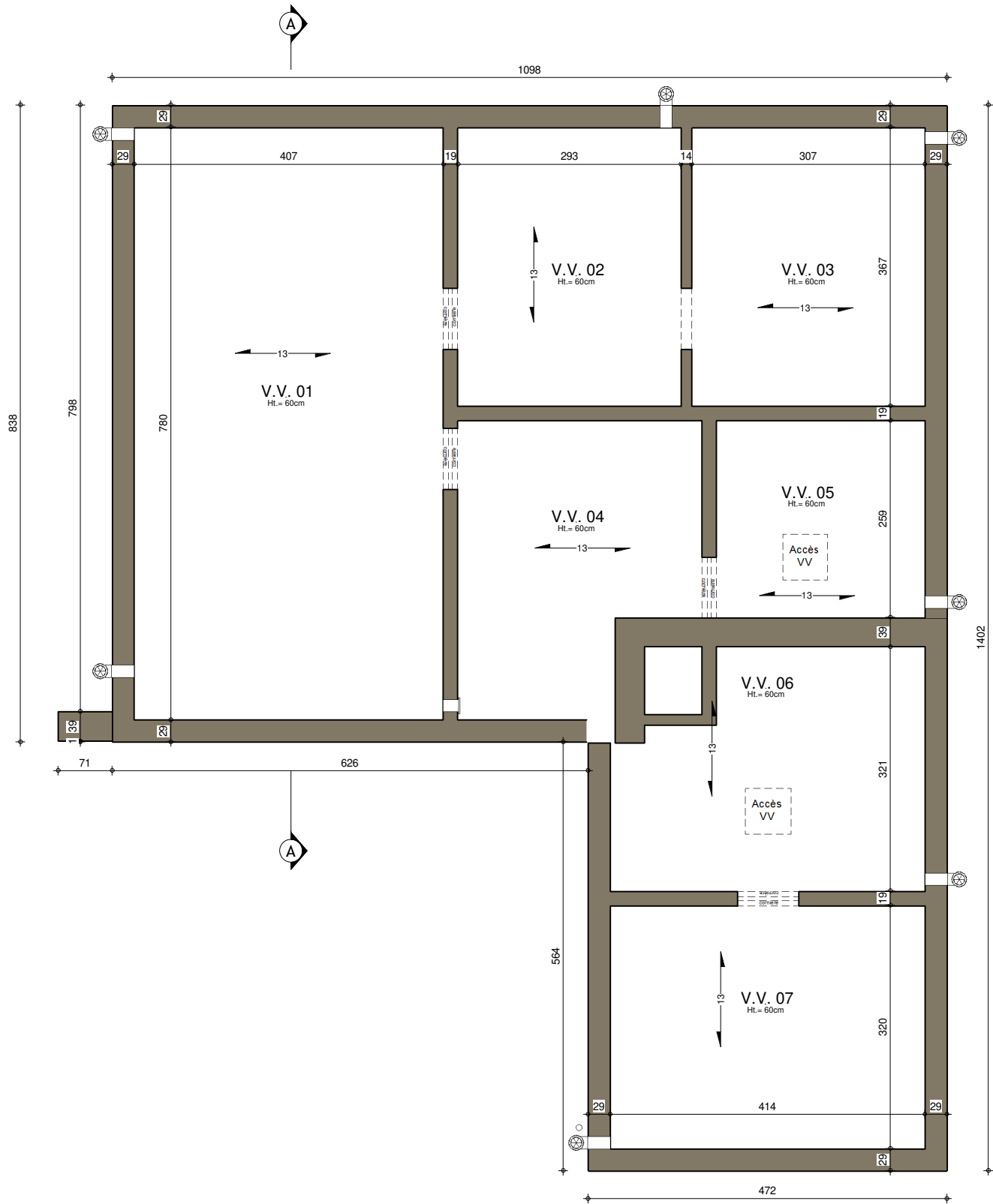
SOUS-SOL : Egouttage
