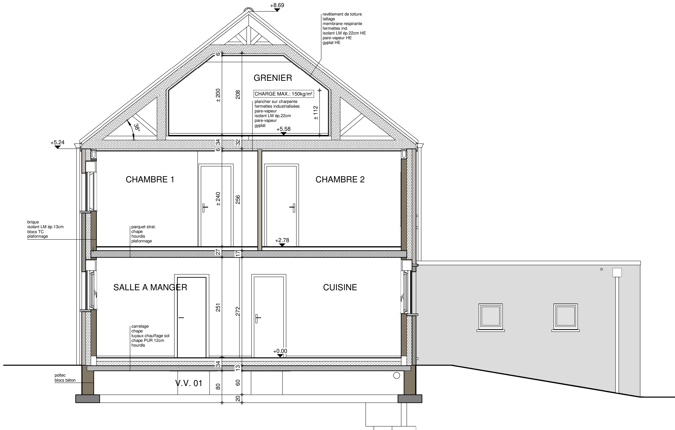
COUPE AA
