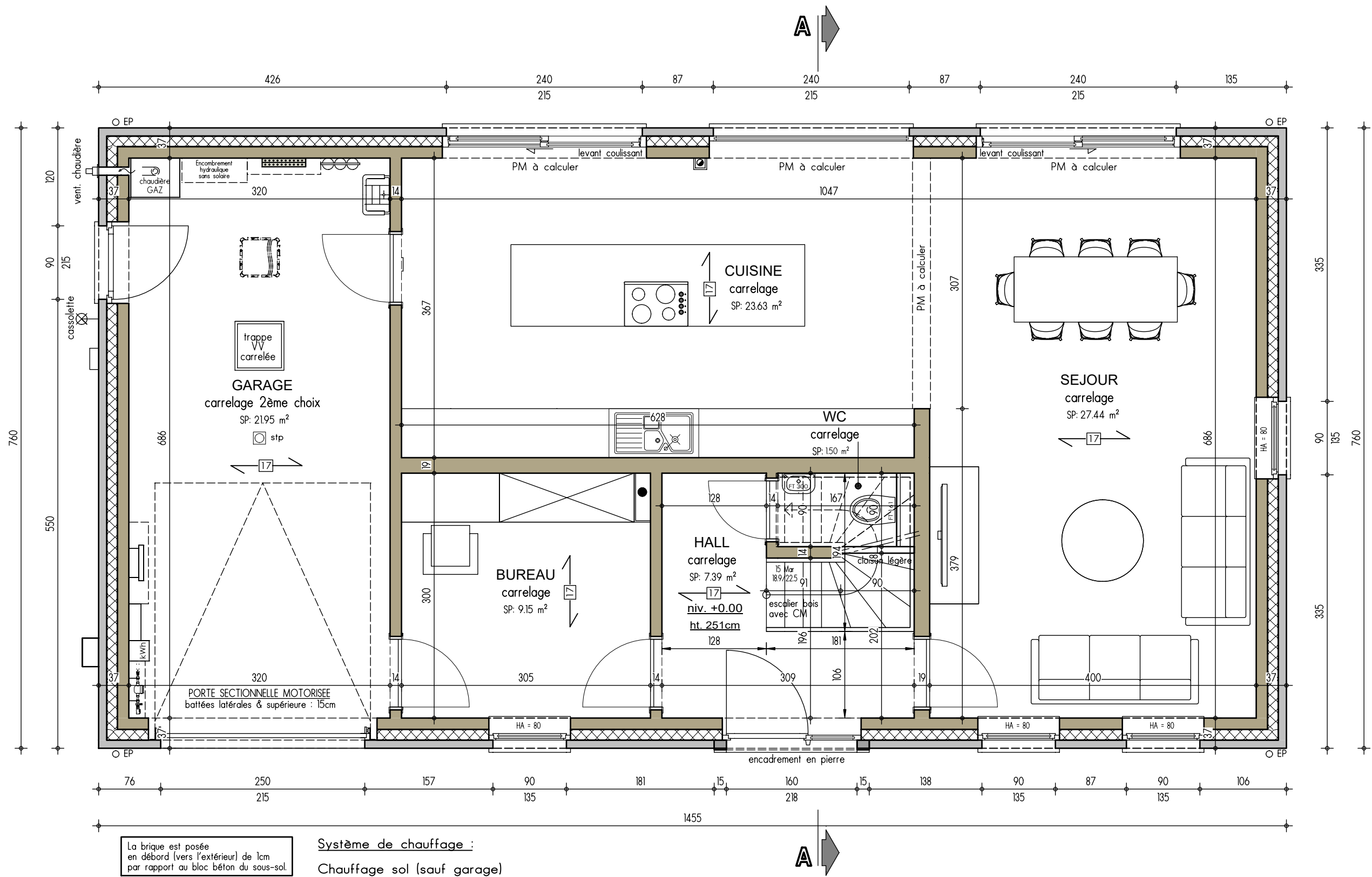
PLAN REZ-DE-CHAUSSE
