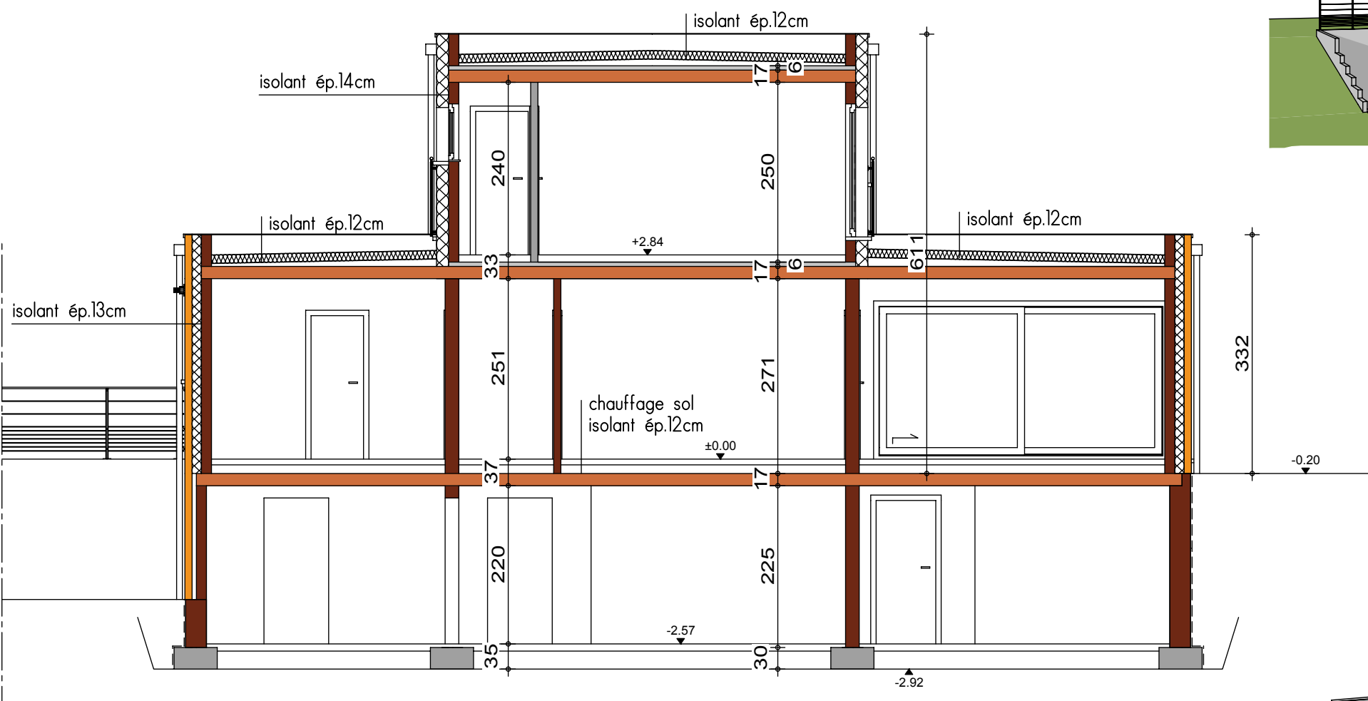
COUPE AA
