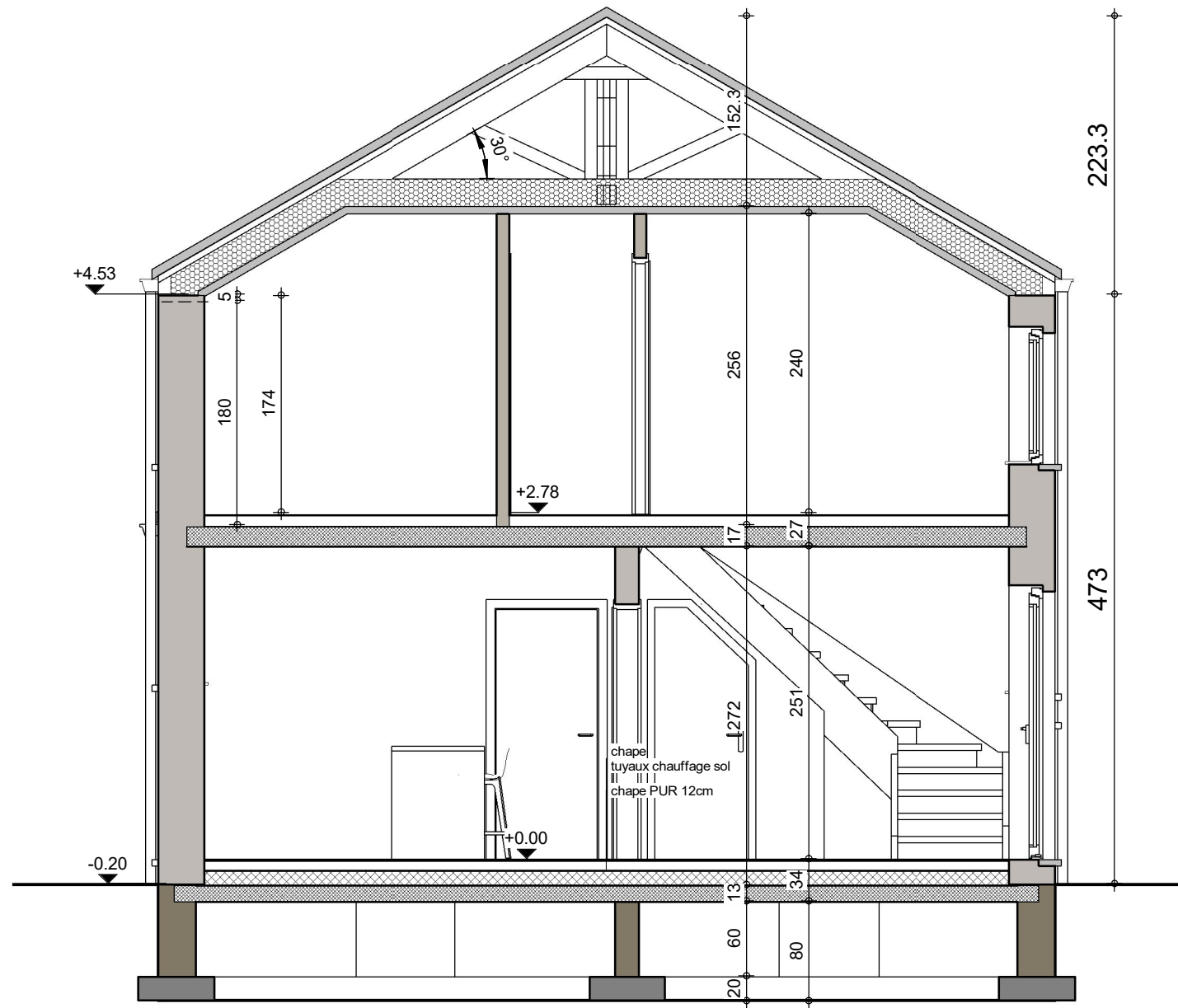
COUPE AA
