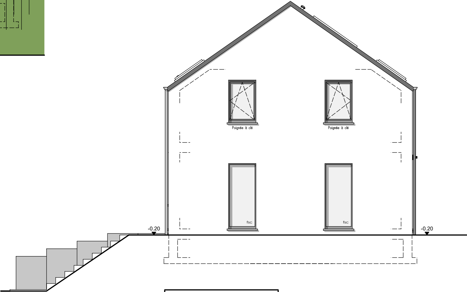
PIGNON DROIT
