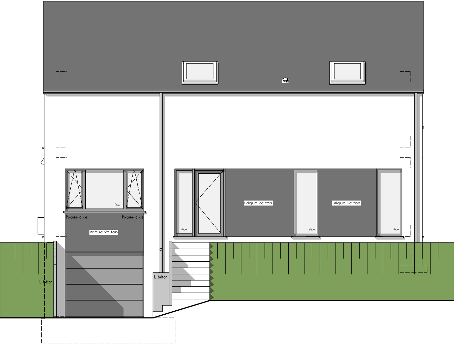
FACADE AVANT
