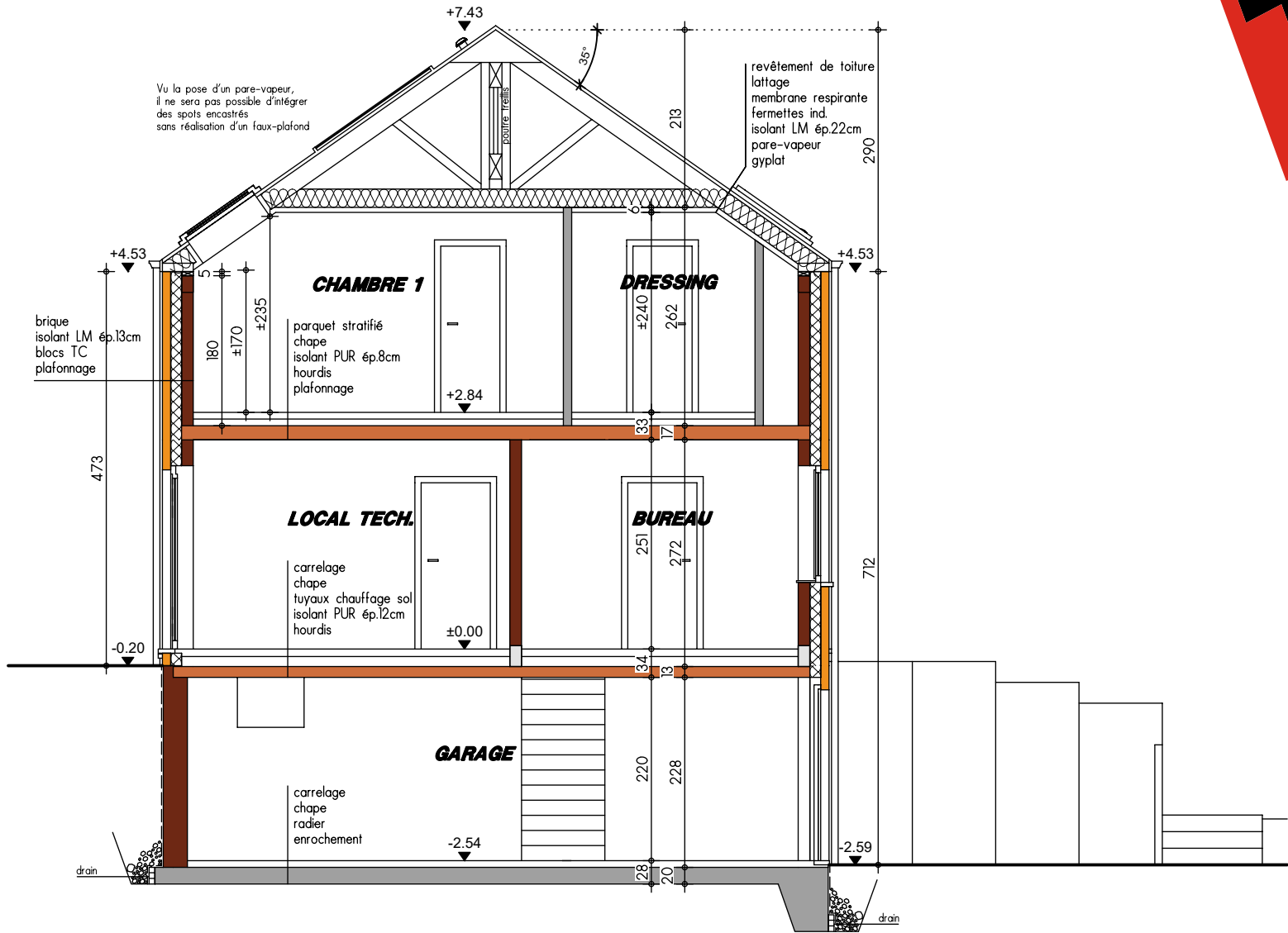
COUPE AA
