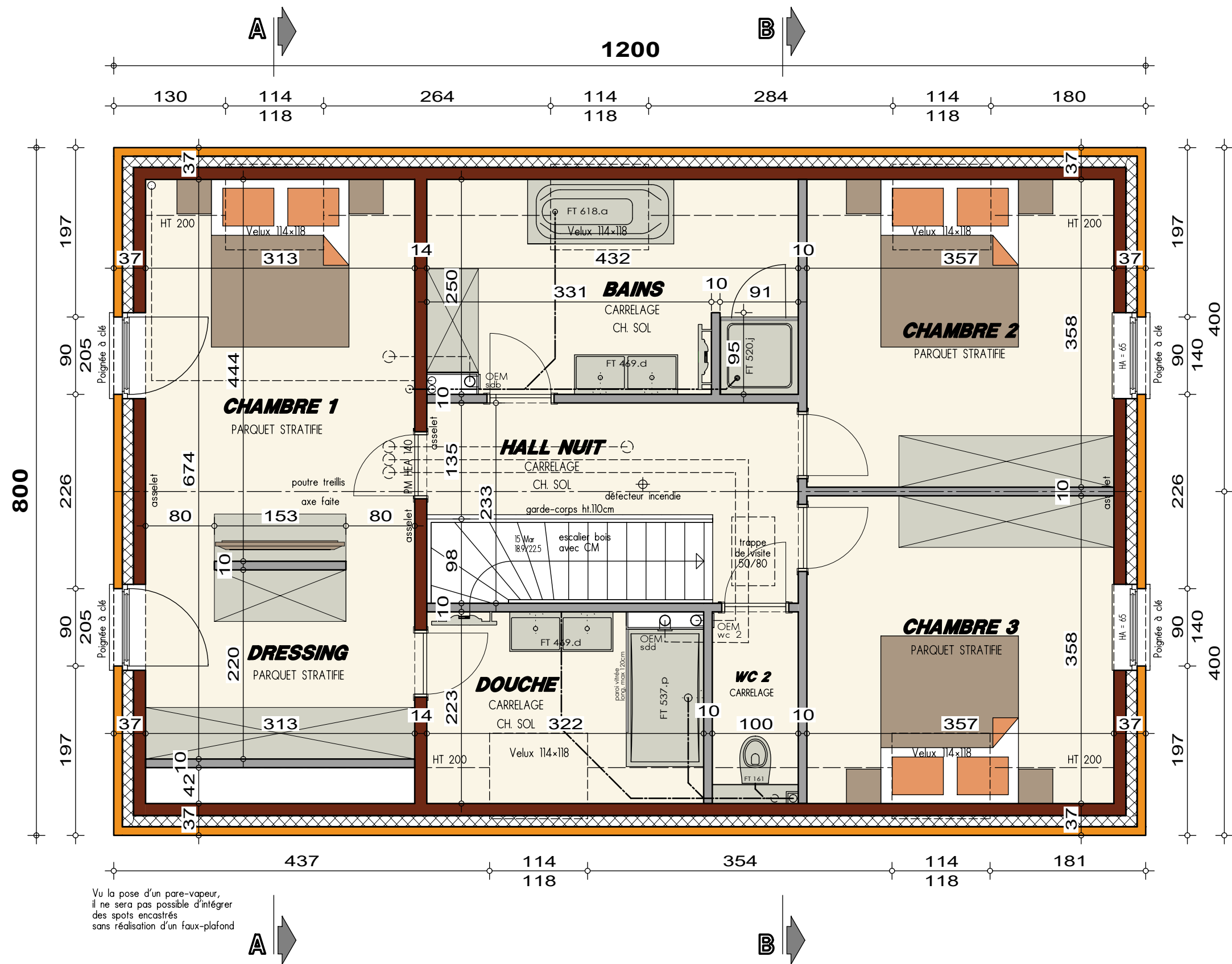
PLAN ETAGE
