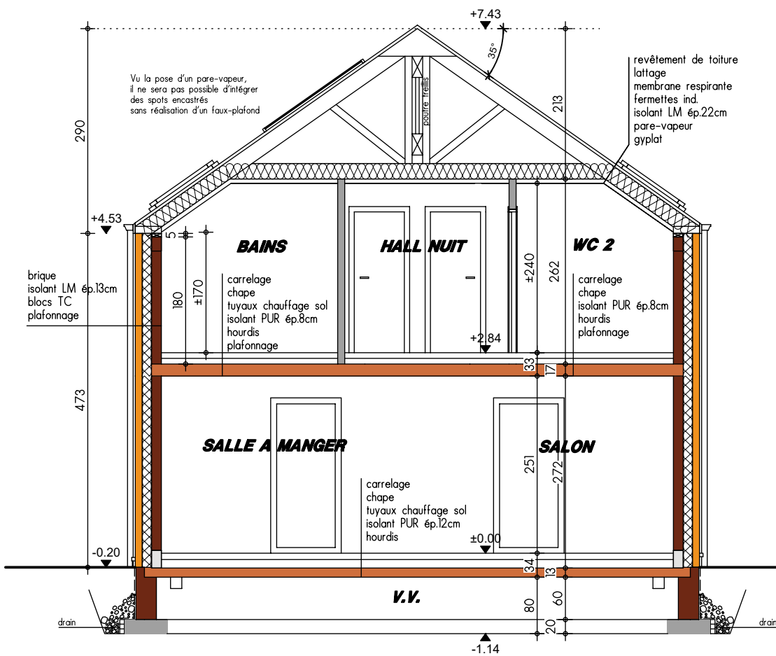
COUPE BB
