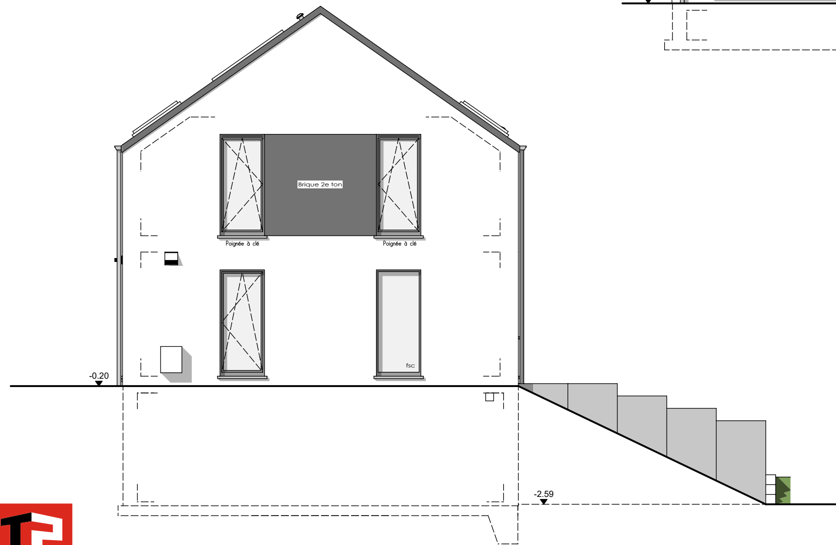
PIGNON GAUCHE
