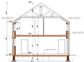
COUPE AA
