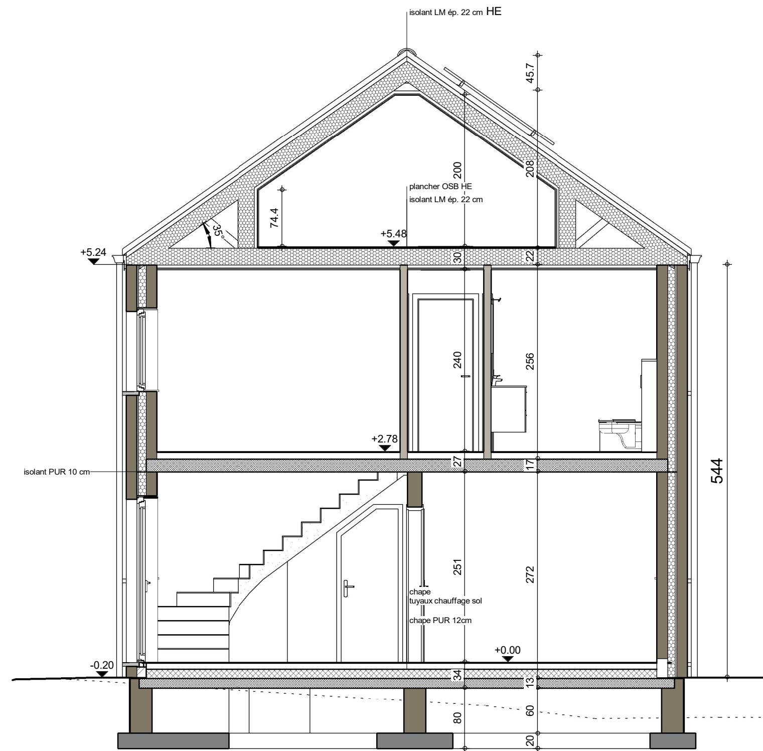
COUPE AA
