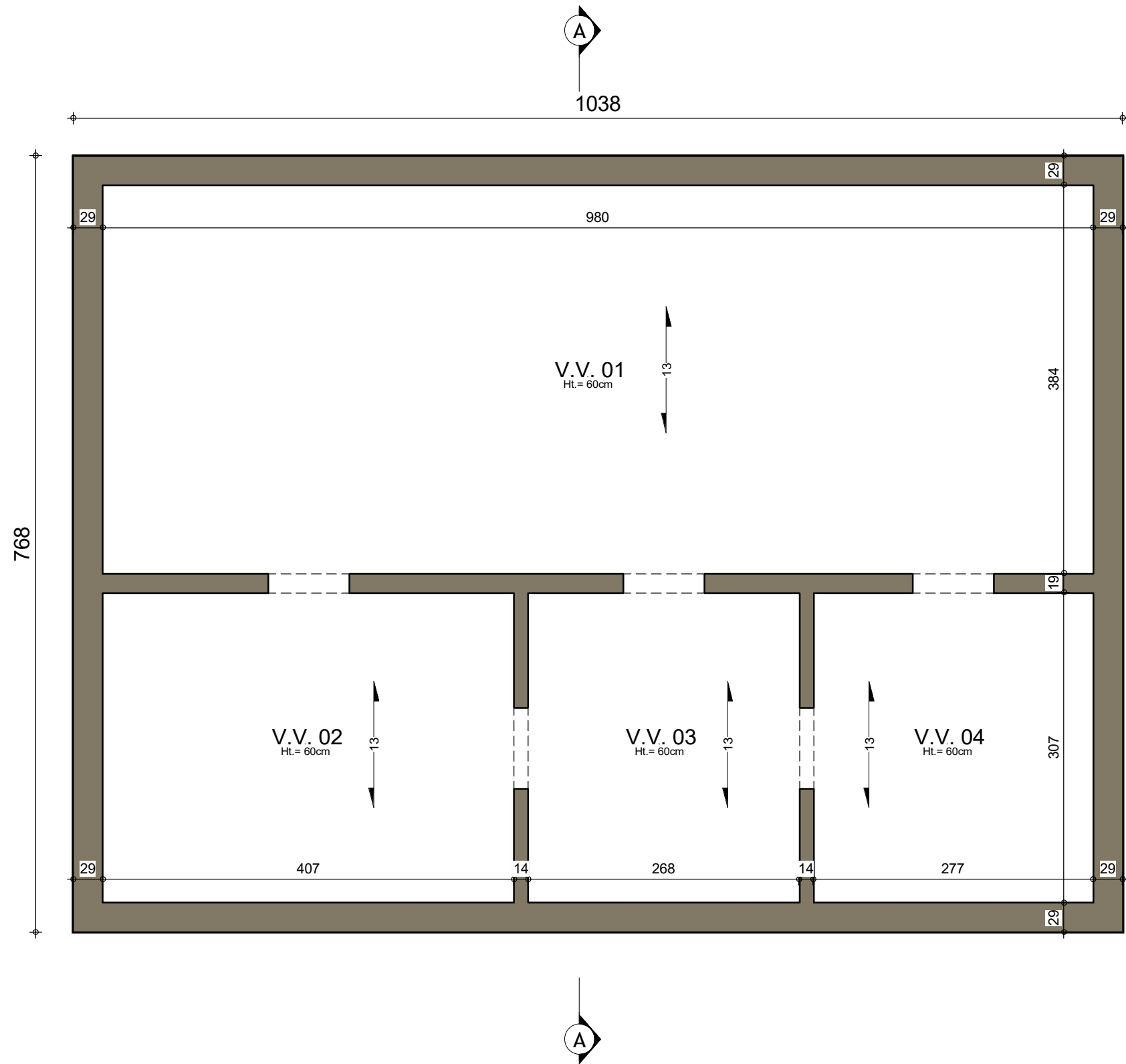
SOUS-SOL
