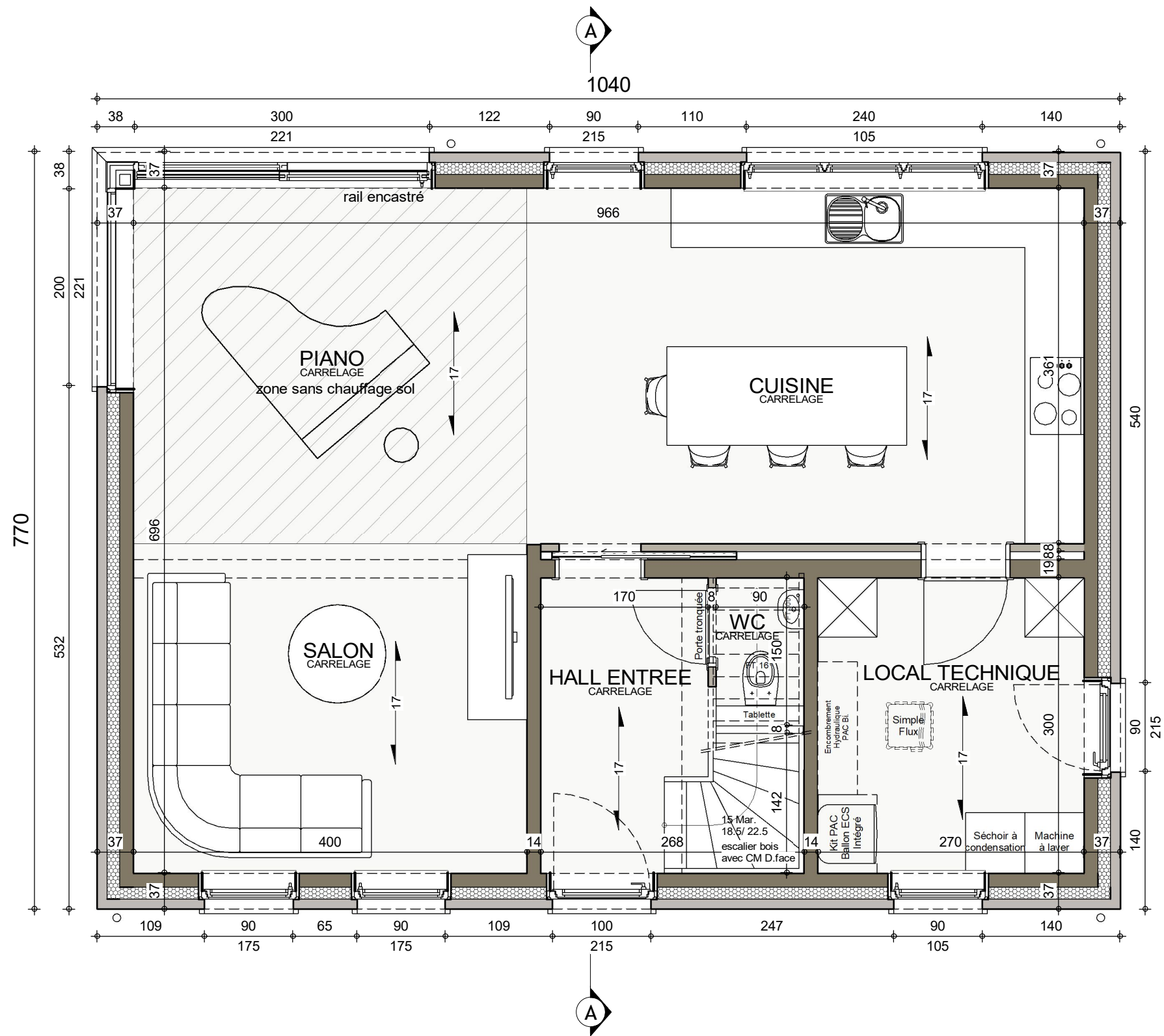
REZ-DE-CHAUSSEE
