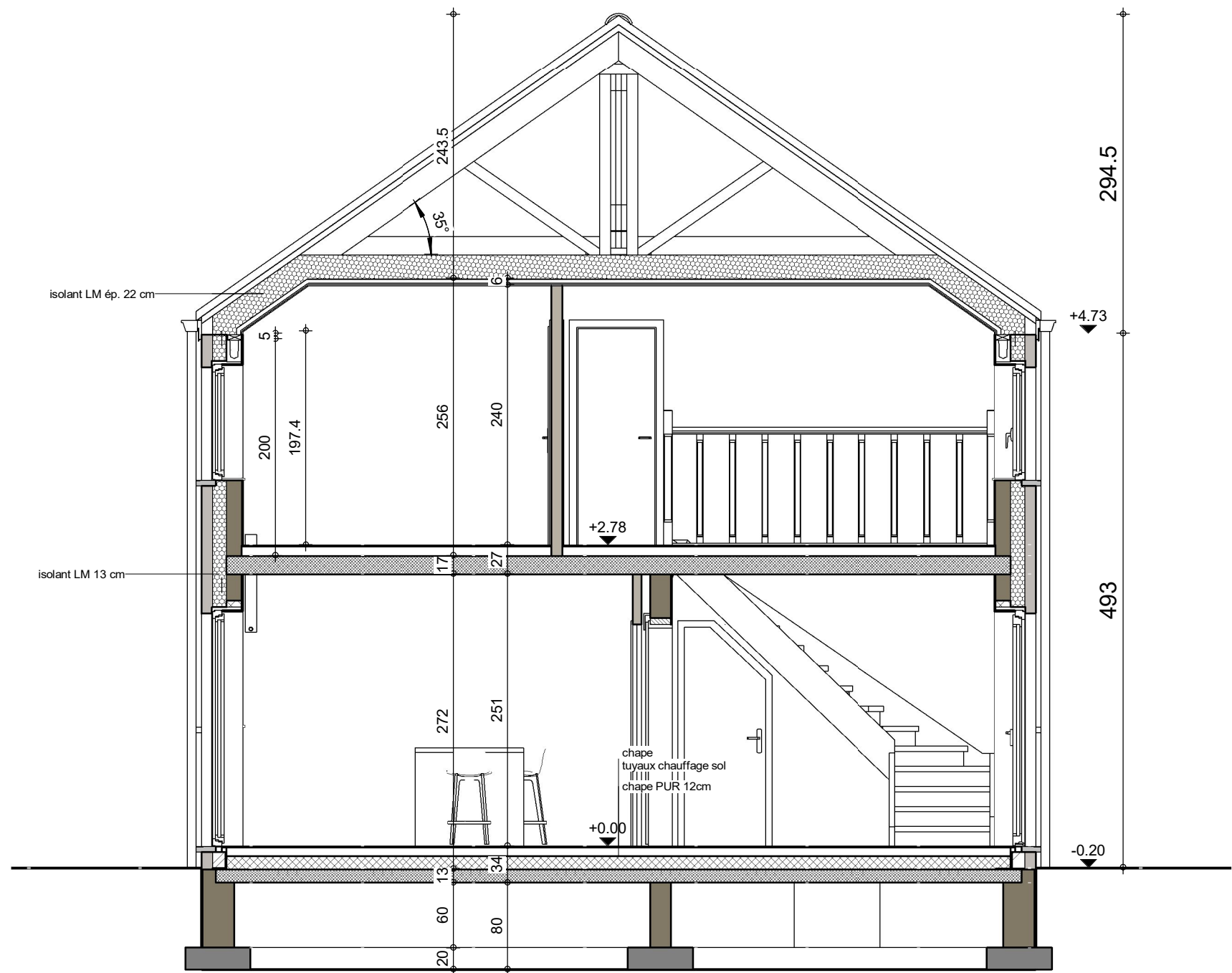
COUPE AA
