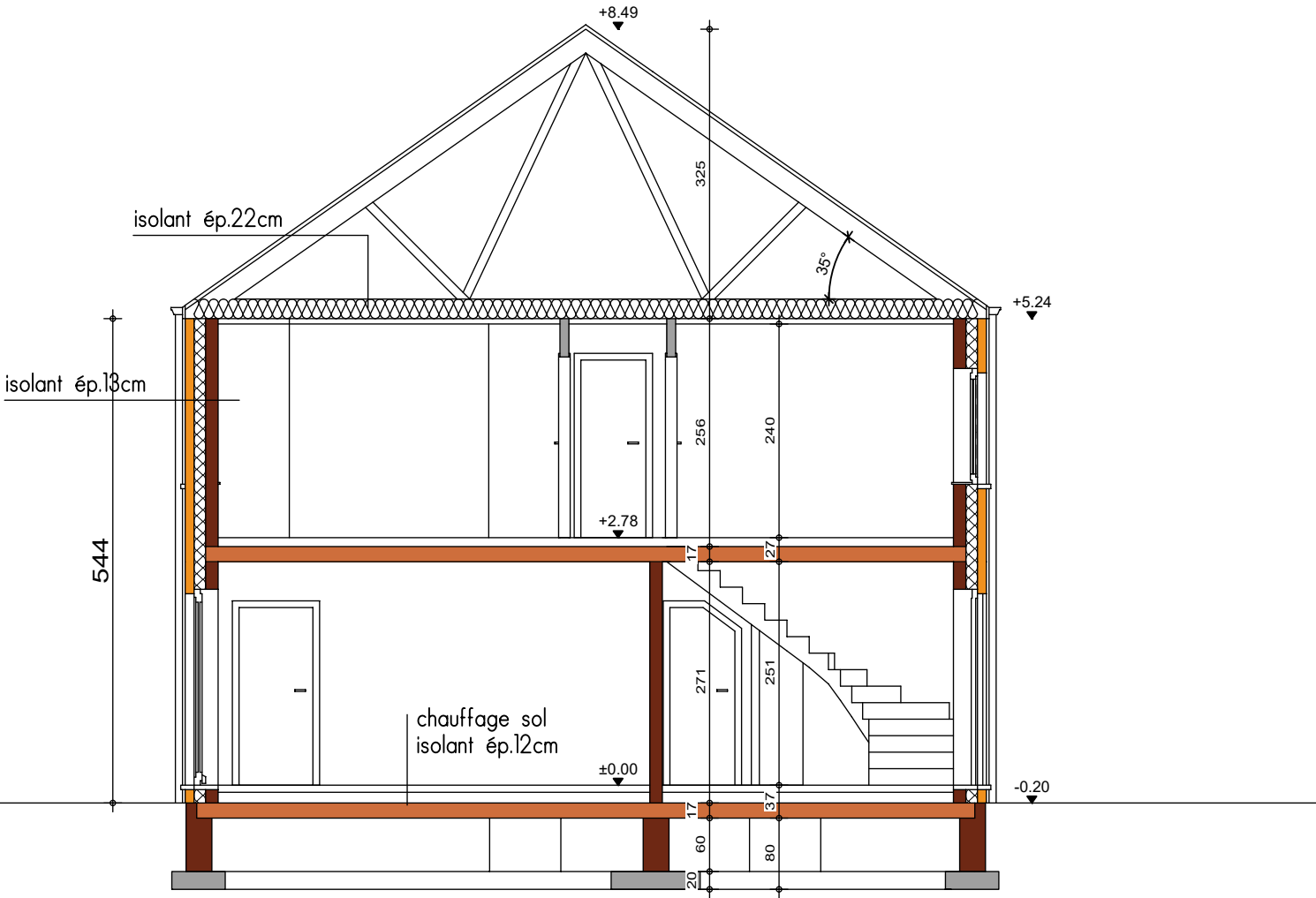
COUPE AA
