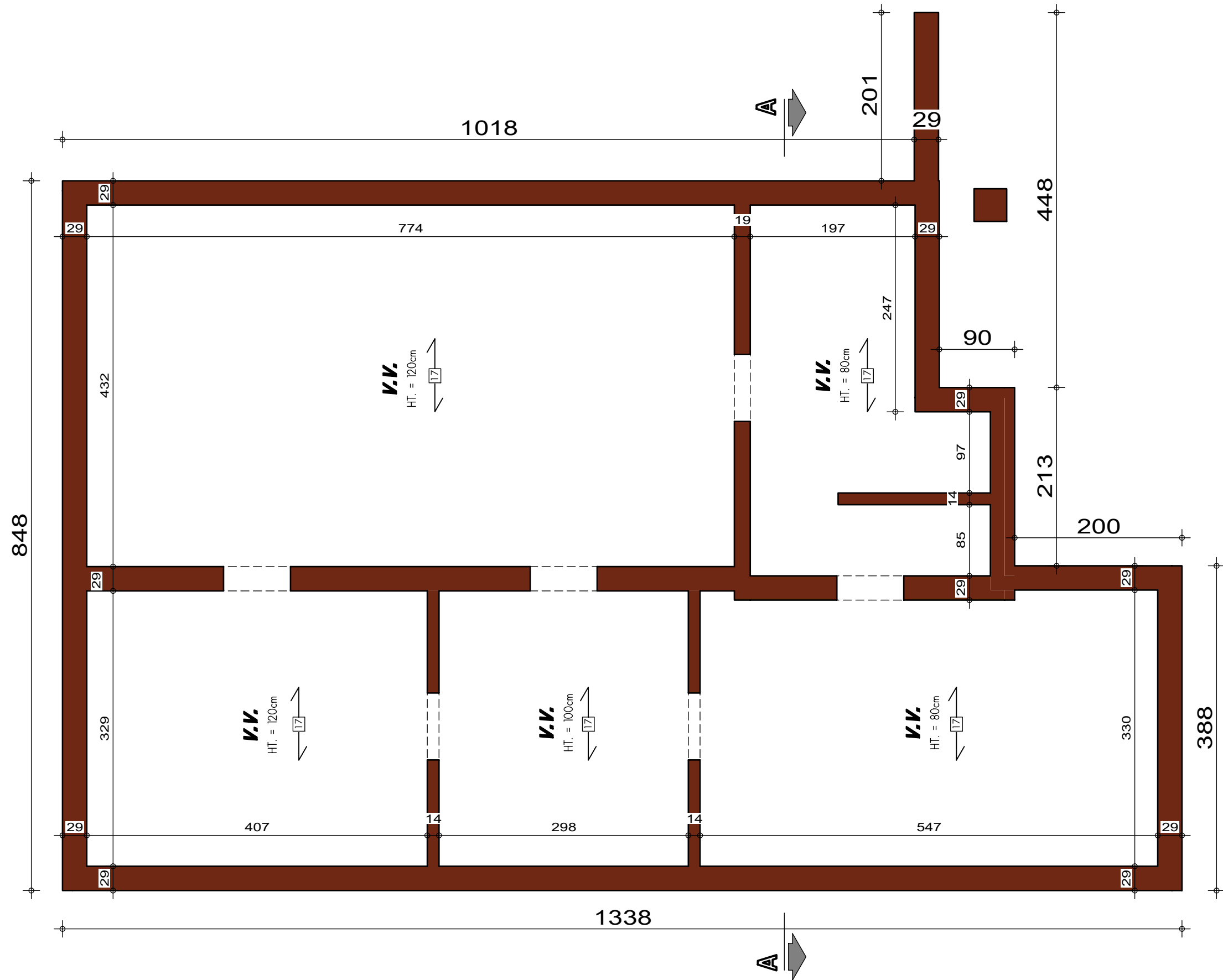
PLAN SOUS-SOL
