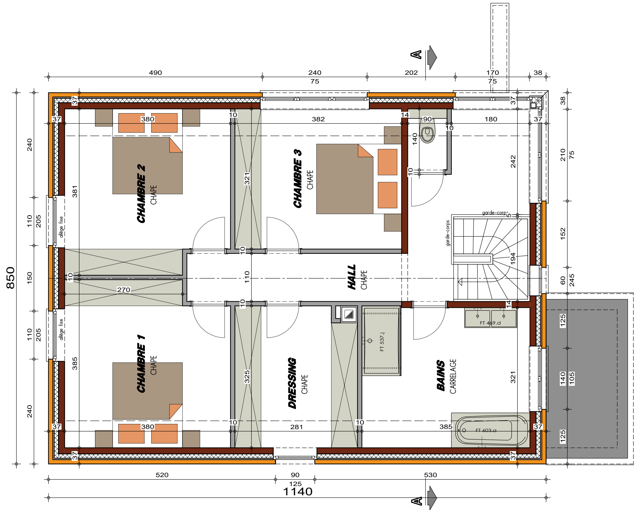
PLAN ETAGE
