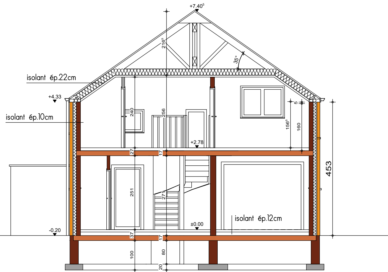
COUPE AA
