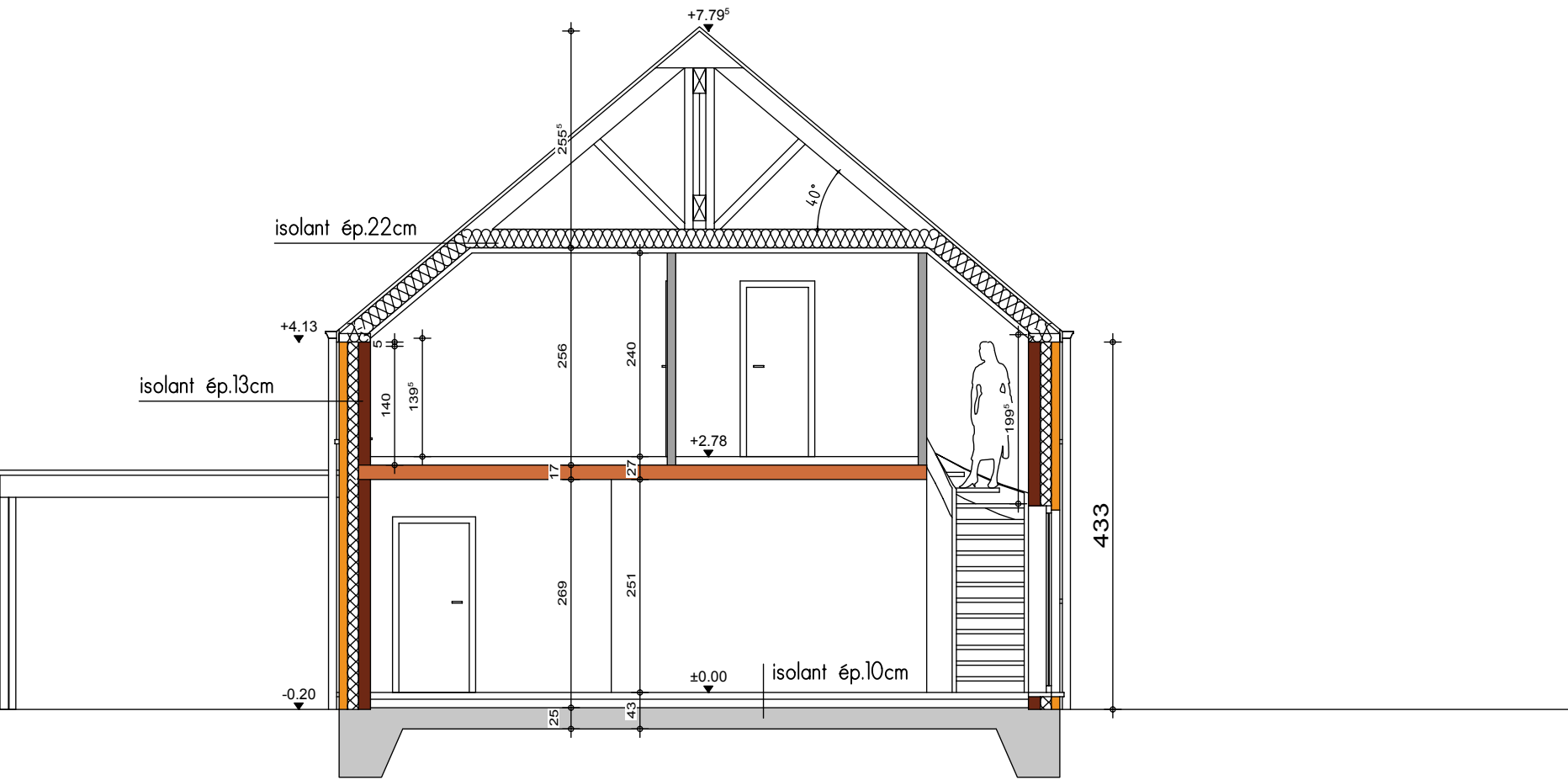
COUPE AA
