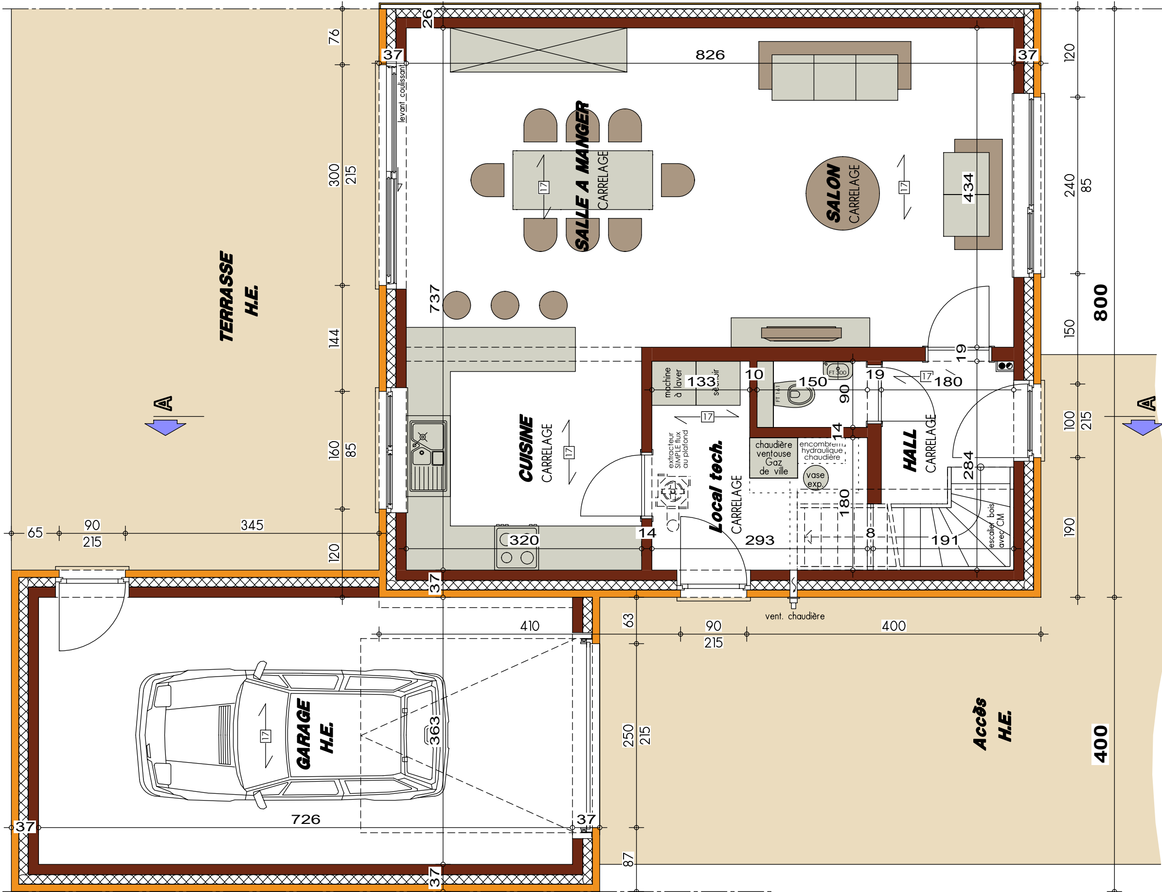
PLAN REZ-DE-CHAUSSEE
