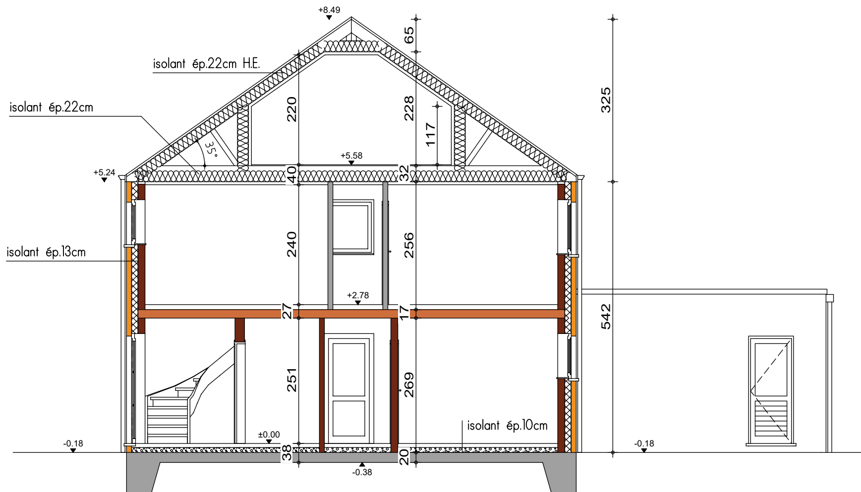
COUPE AA
