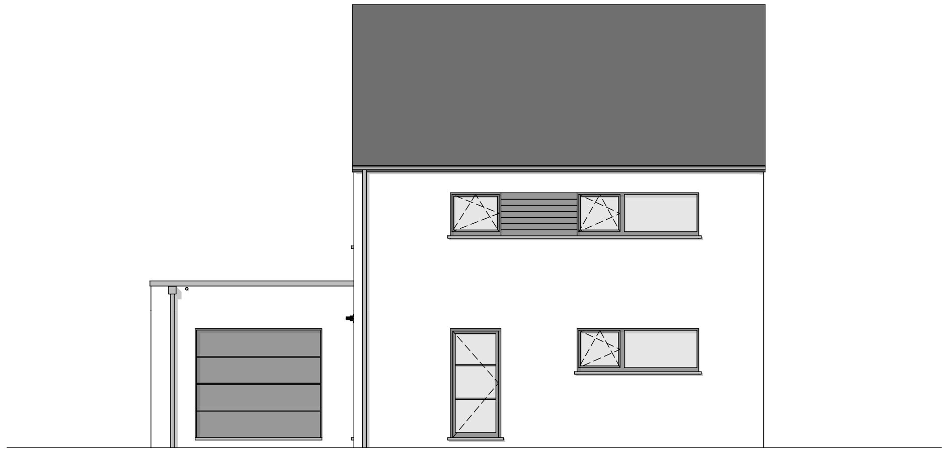
FACADE AVANT
