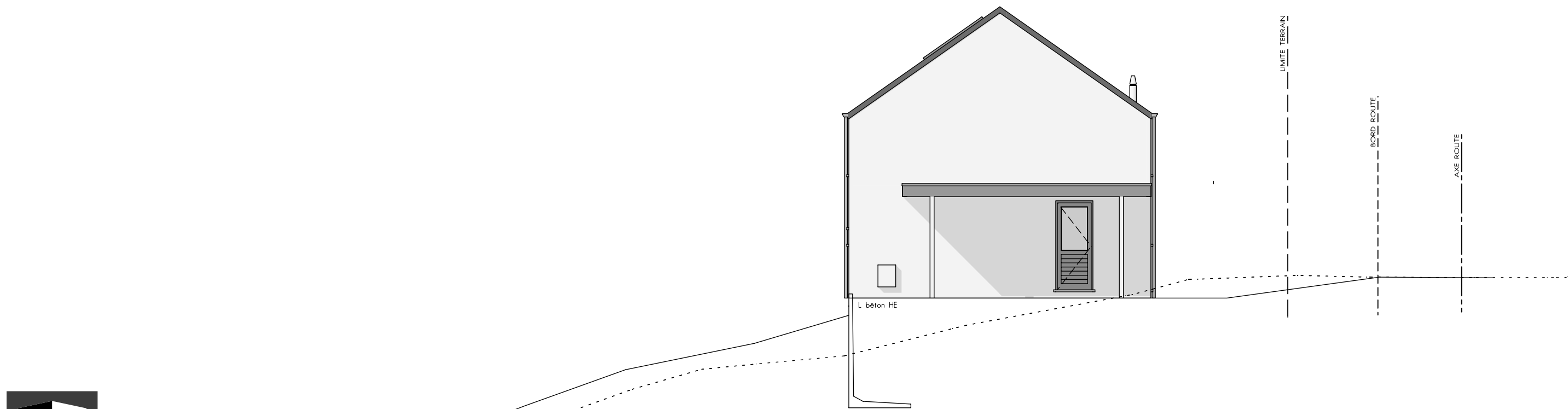
PIGNON GAUCHE
