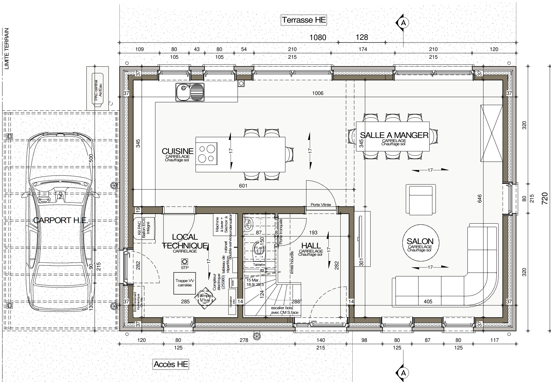
REZ-DE-CHAUSSEE
