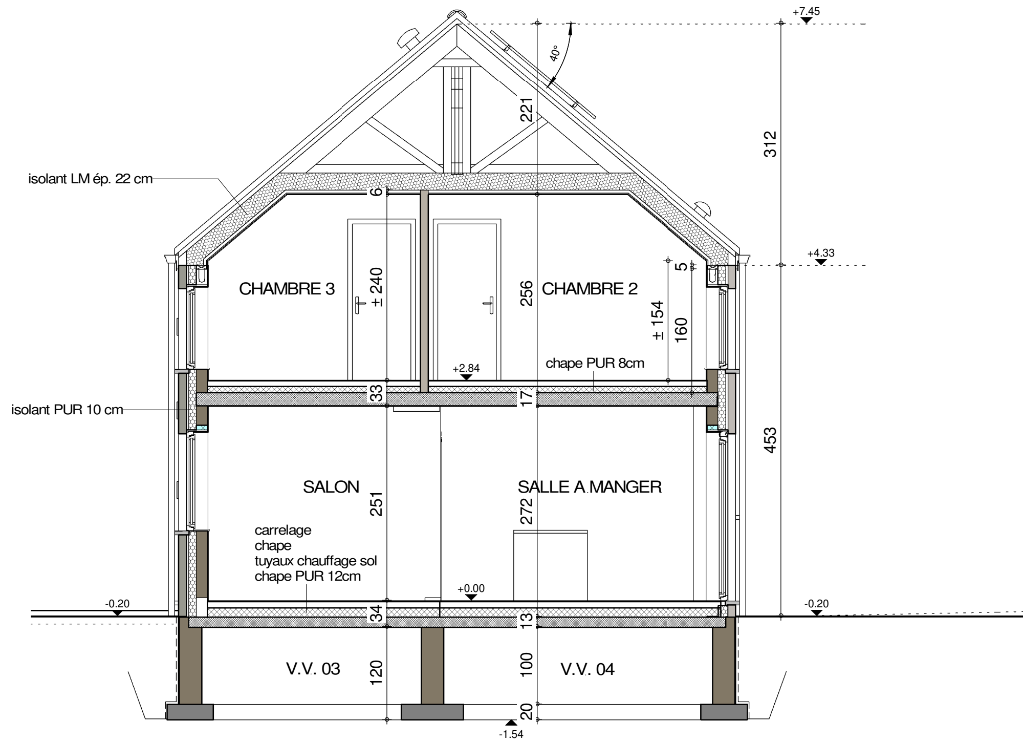
COUPE AA
