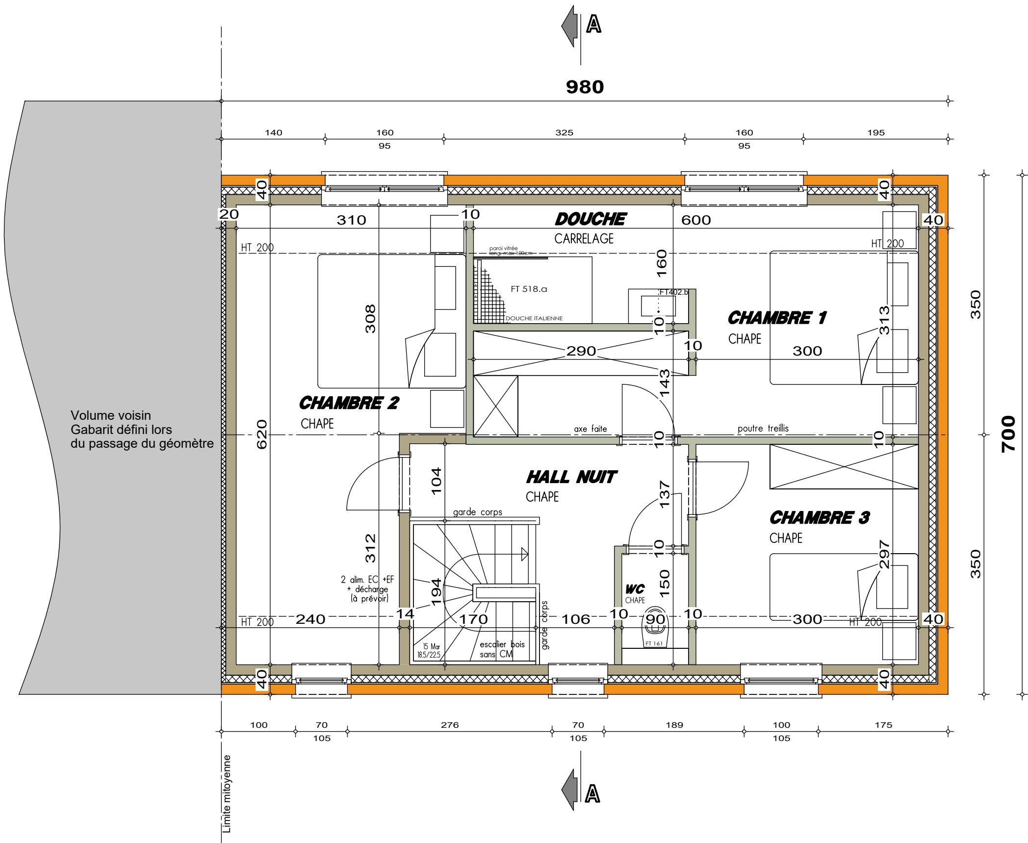
PLAN ETAGE
