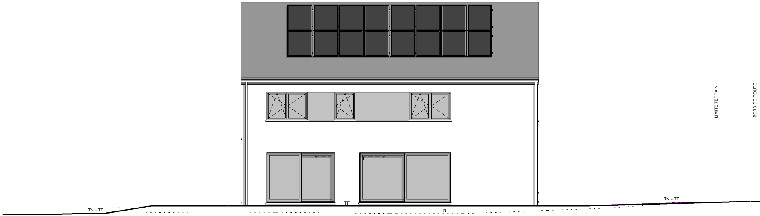
FACADE LATERALE GAUCHE
