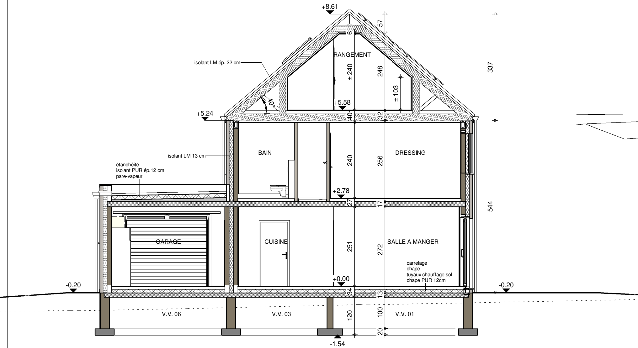
COUPE AA
