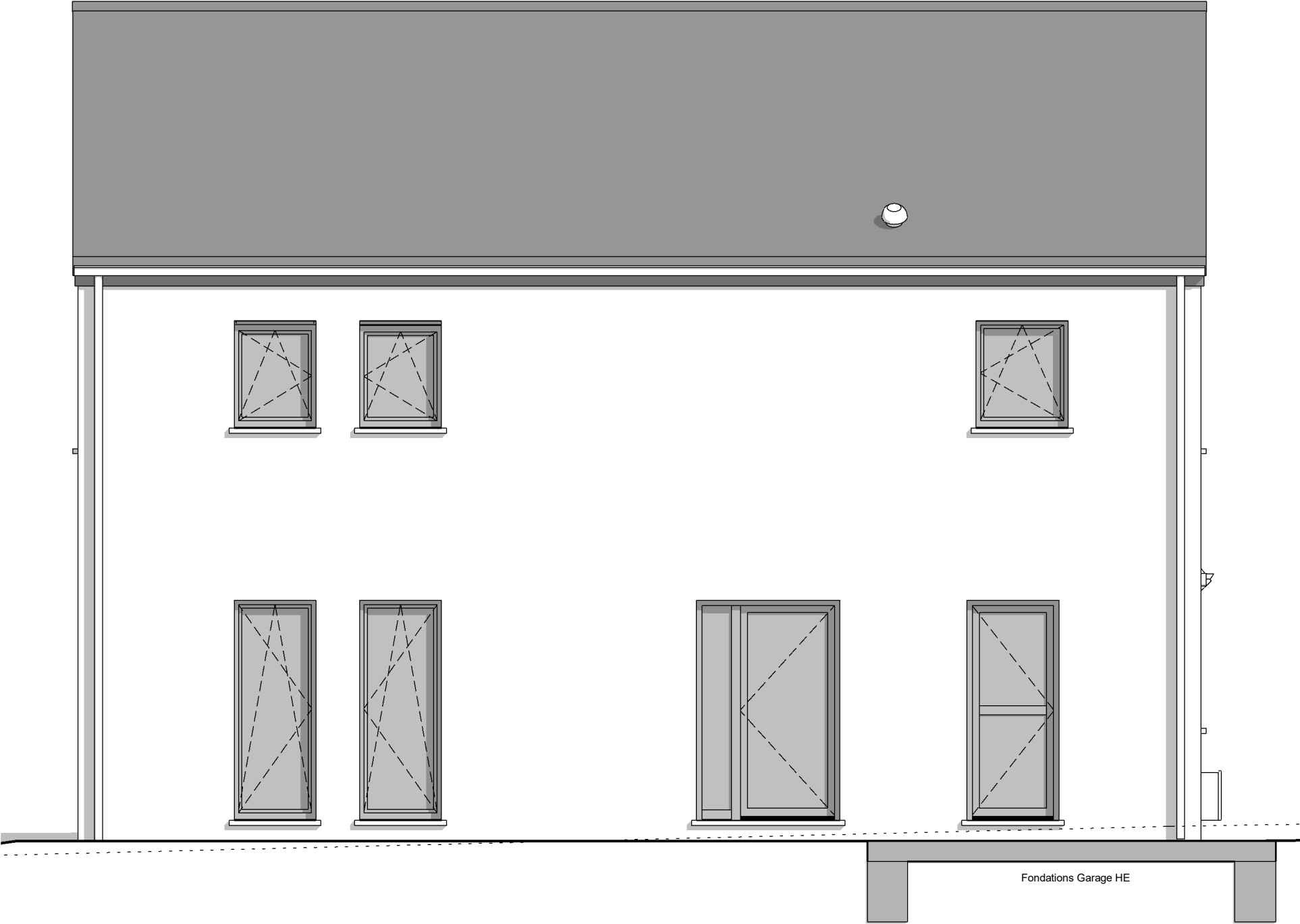
FACADE AVANT
