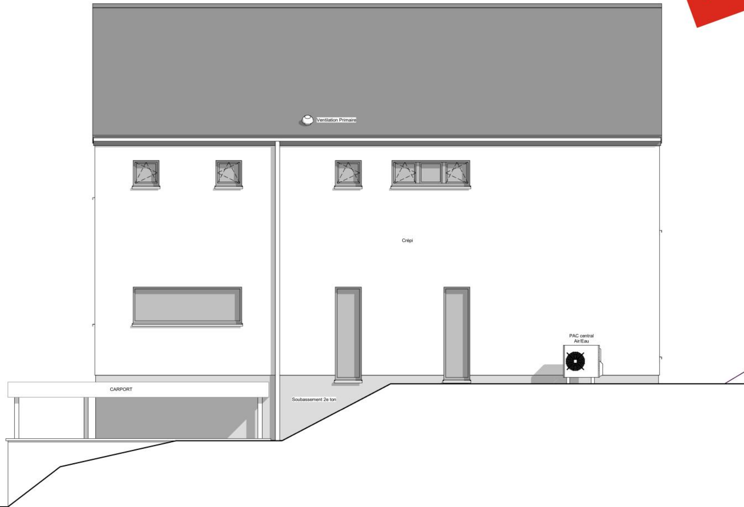
FACADE DROIT
