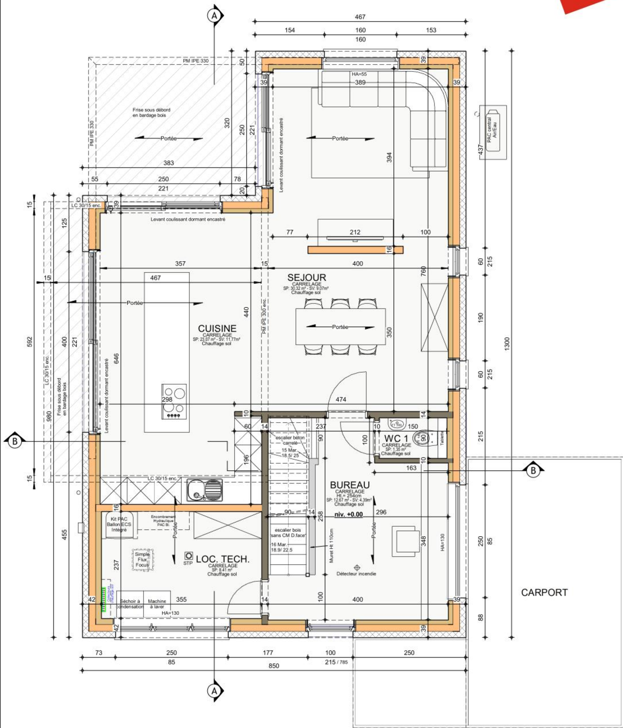
REZ-DE-CHAUSSEE
