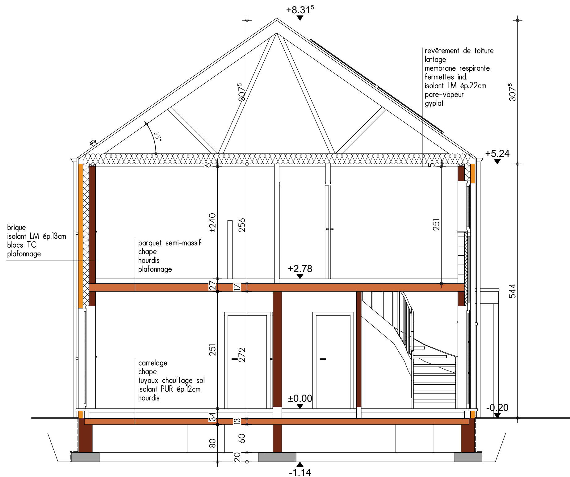
COUPE AA
