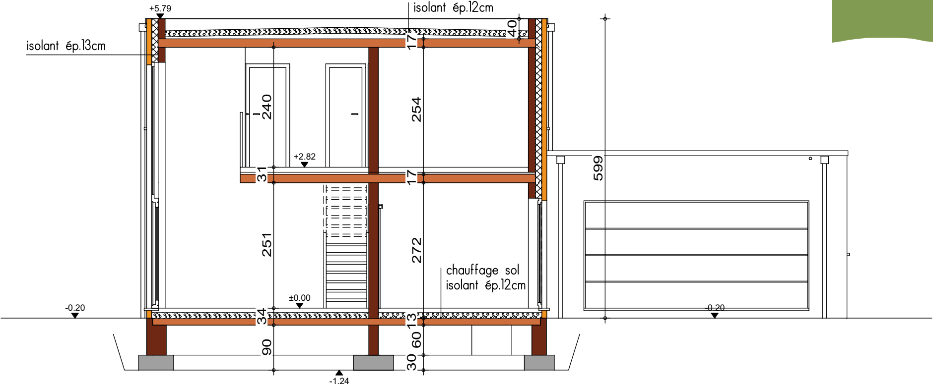
COUPE AA
