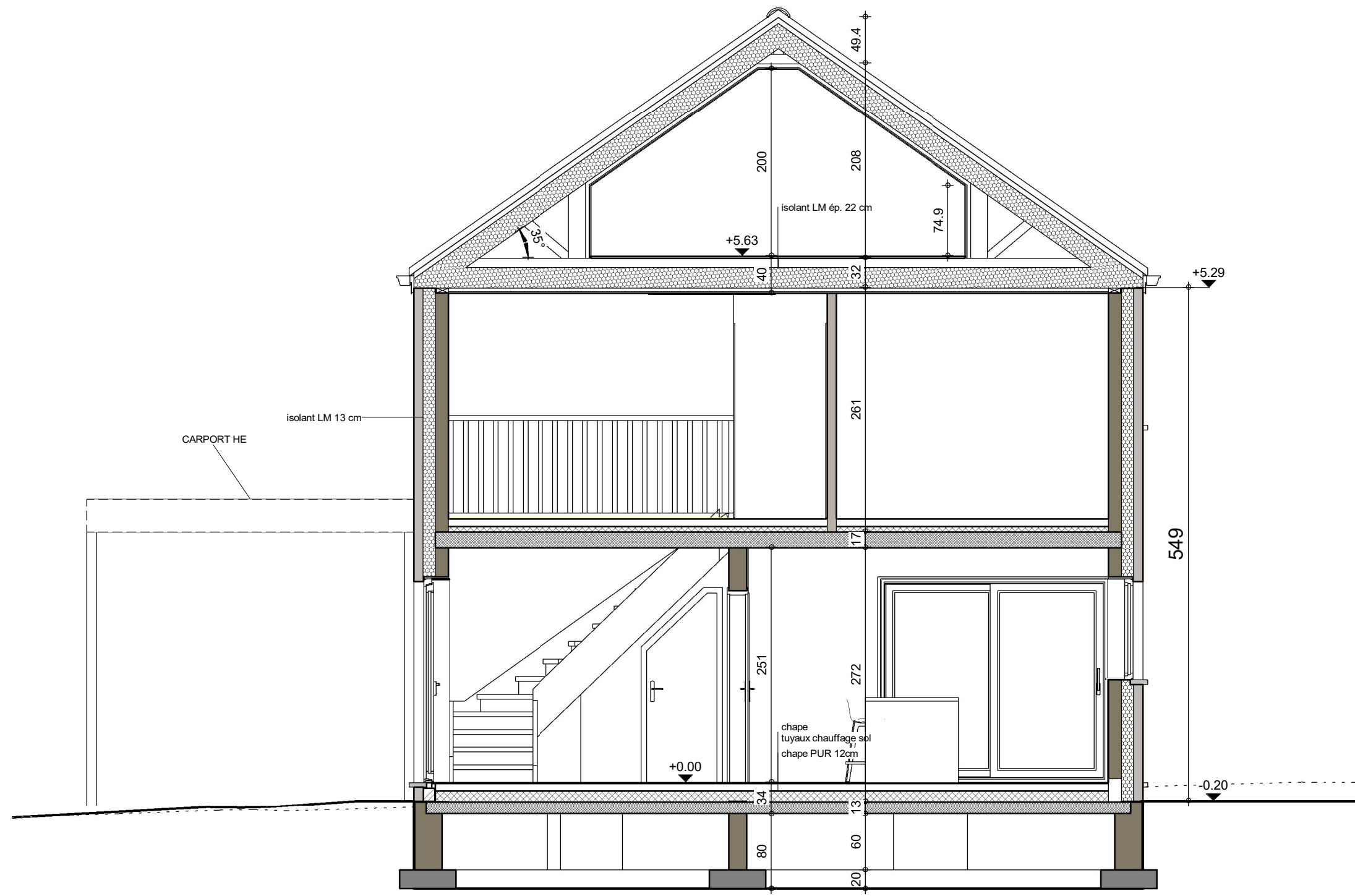
COUPE AA
