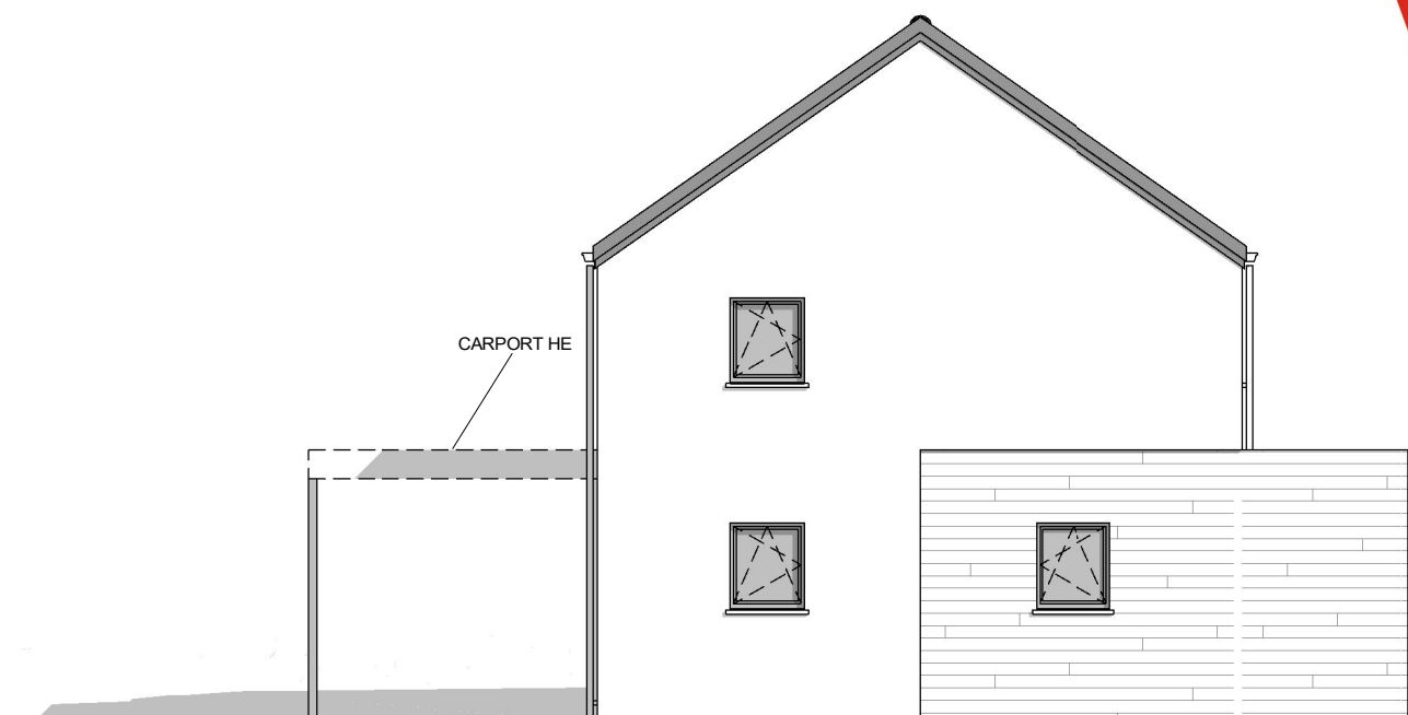
PIGNON DROIT
