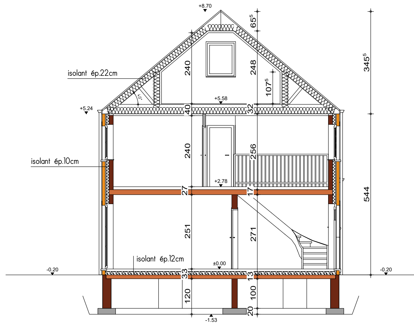
COUPE AA
