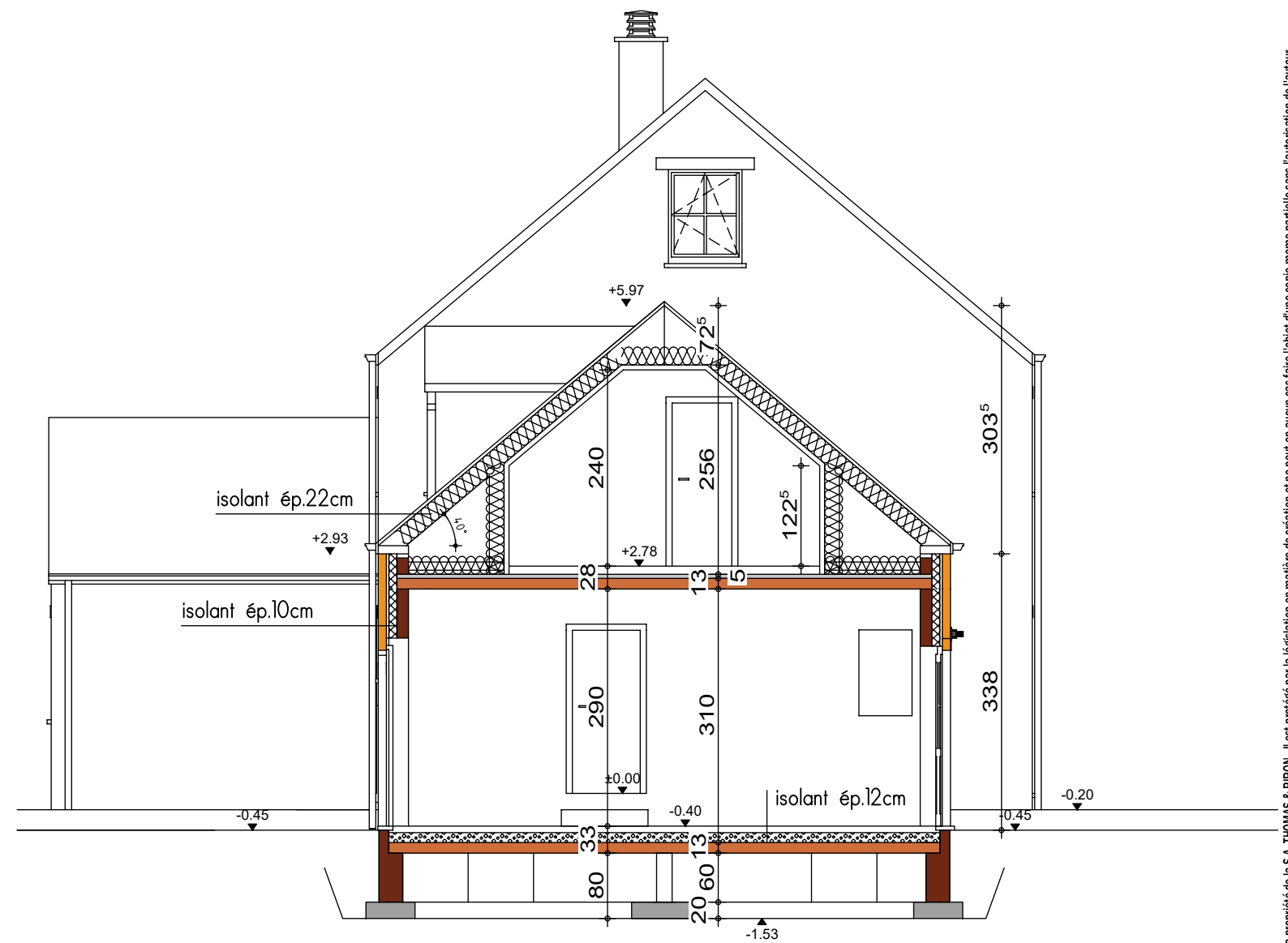
COUPE BB
