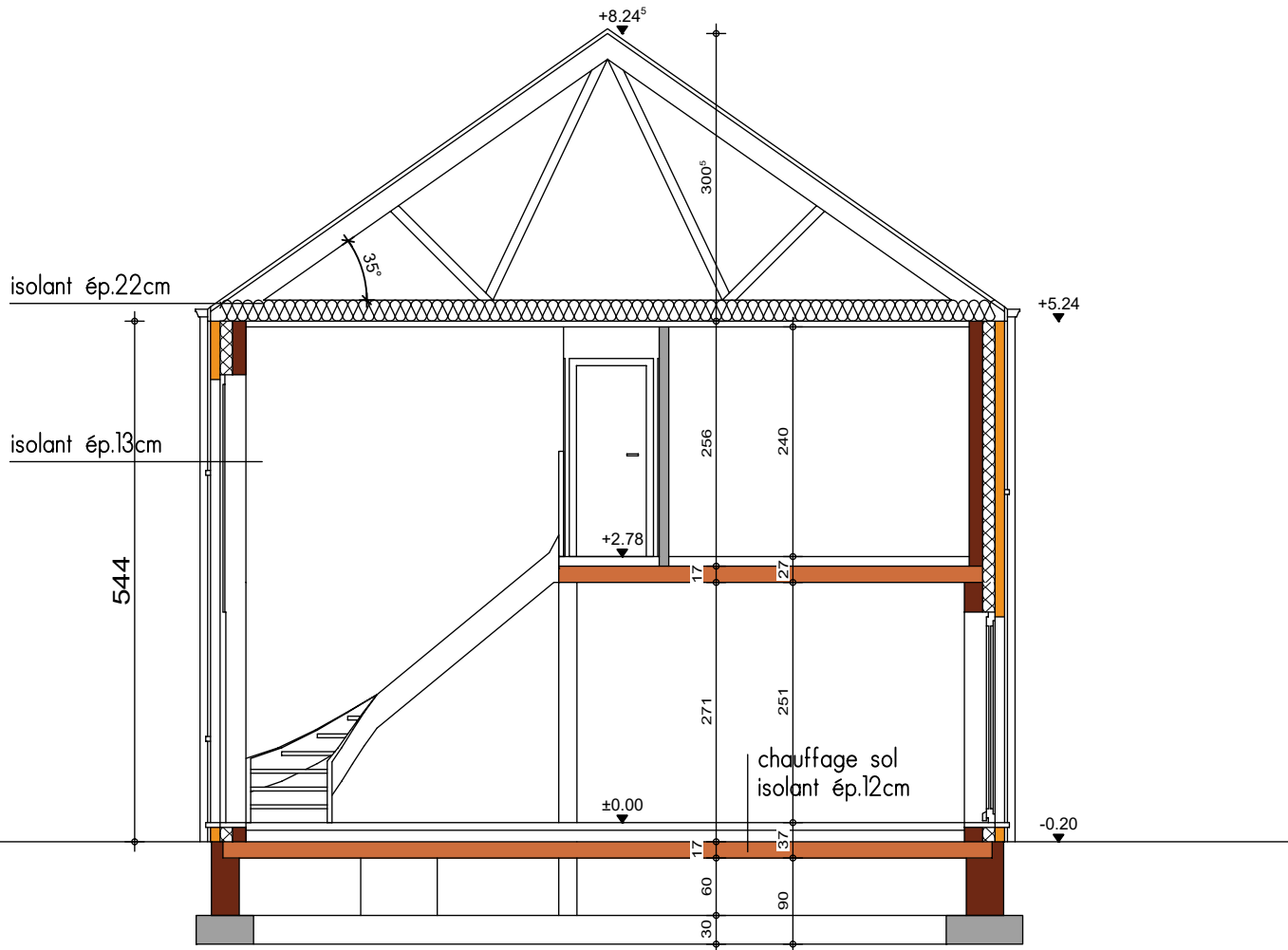
COUPE AA
