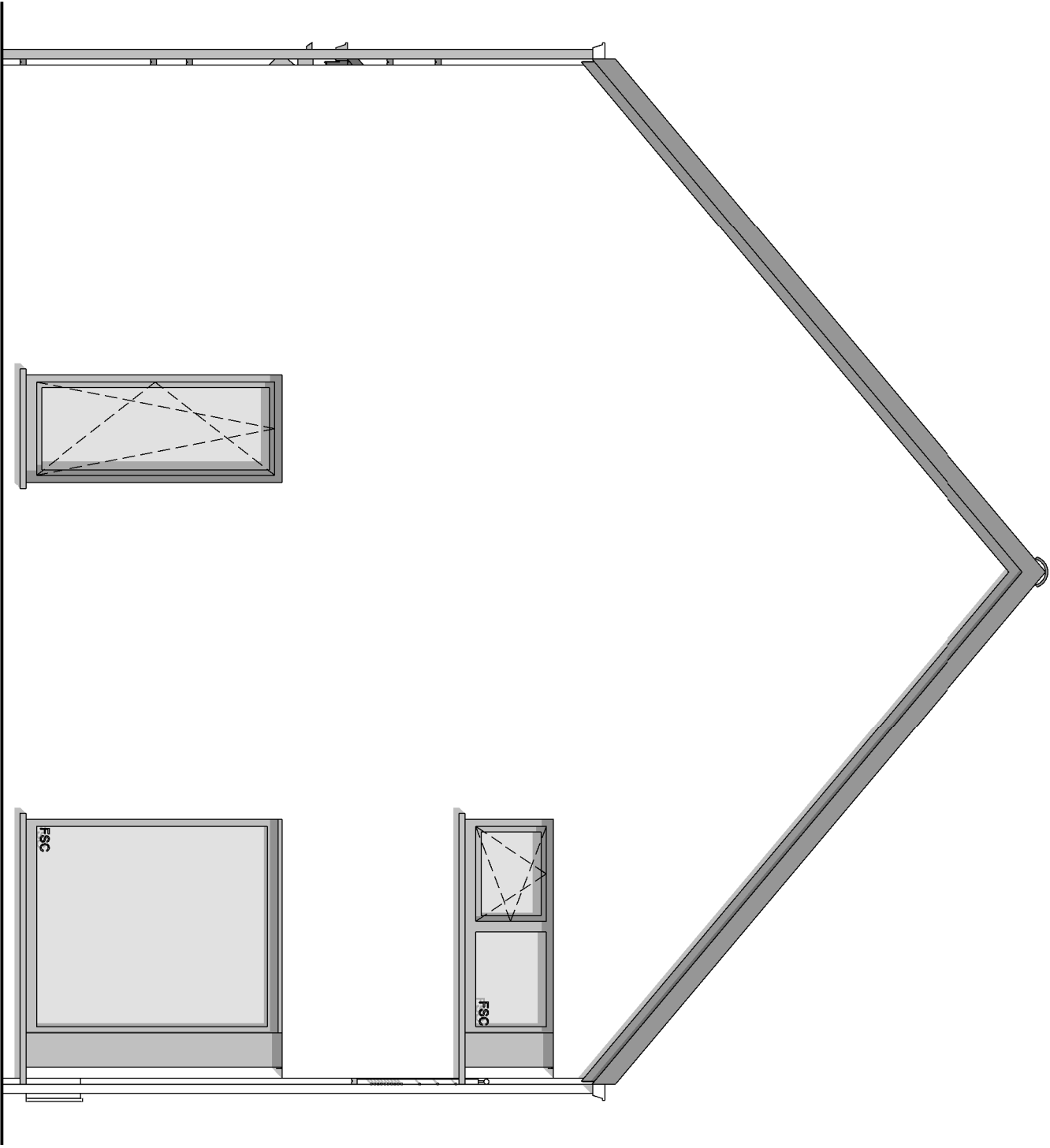
PIGNON GAUCHE
