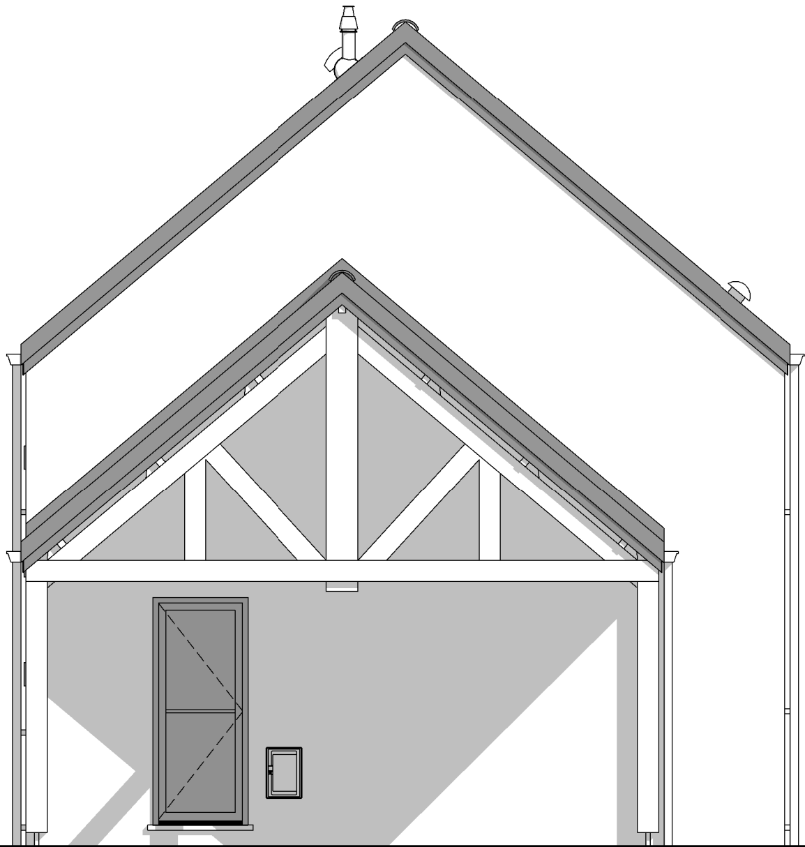
PIGNON DROIT
