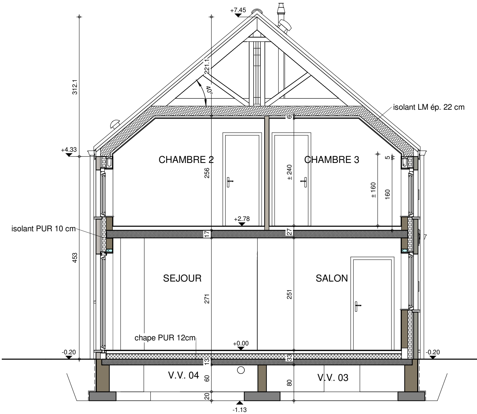
COUPE AA
