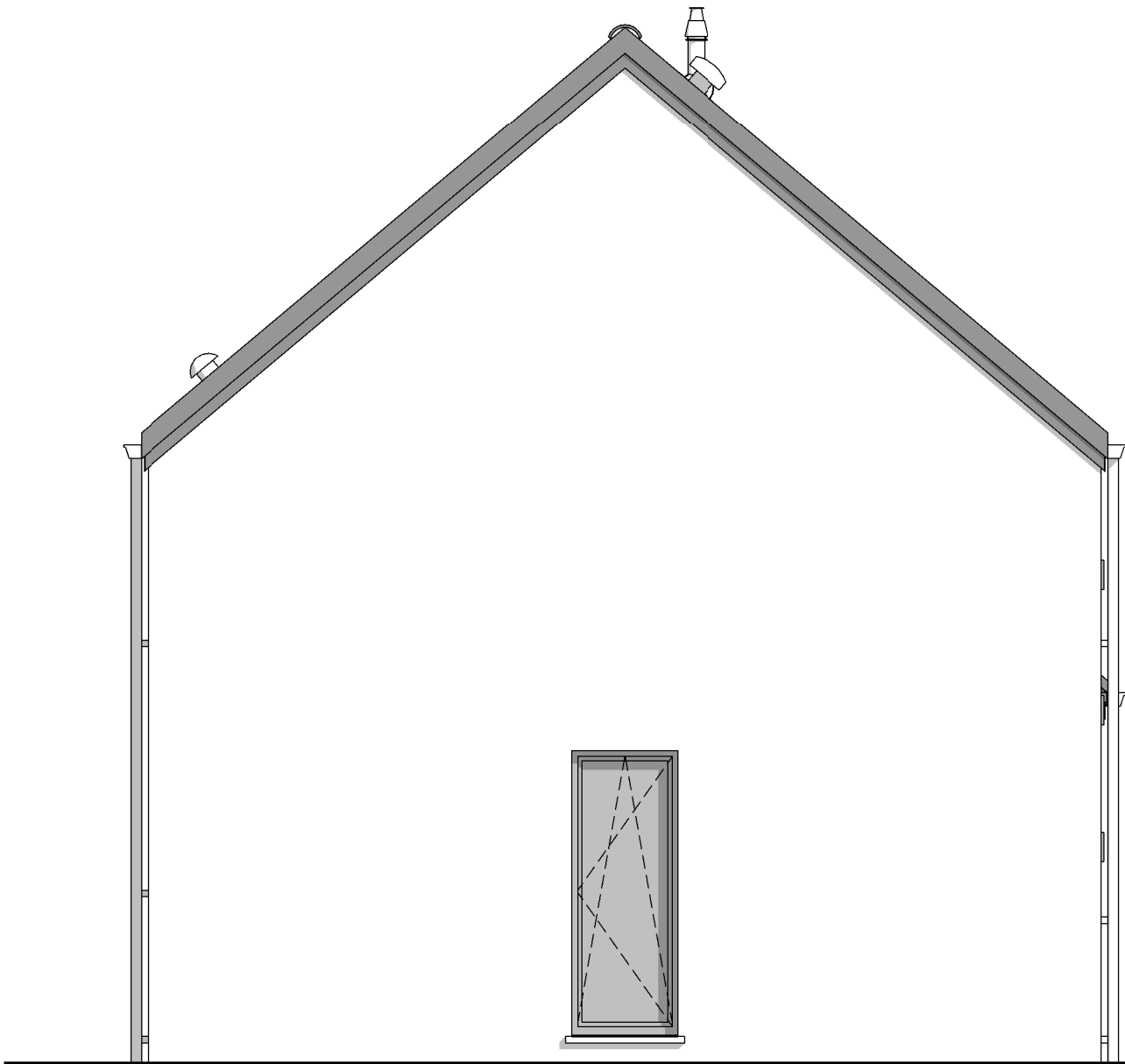
PIGNON GAUCHE
