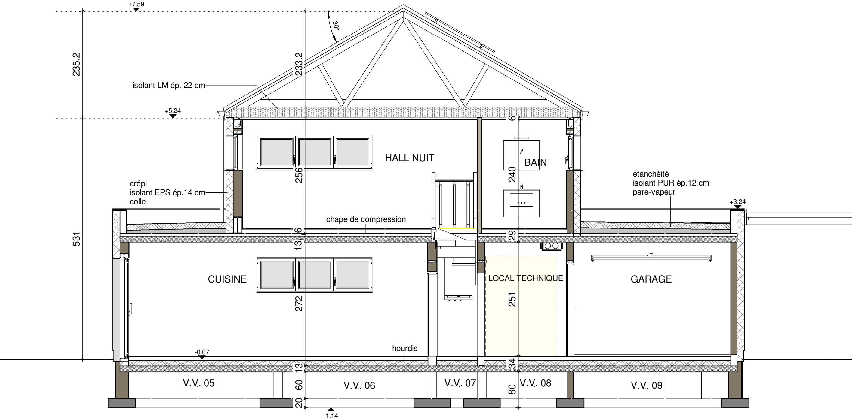
COUPE BB
