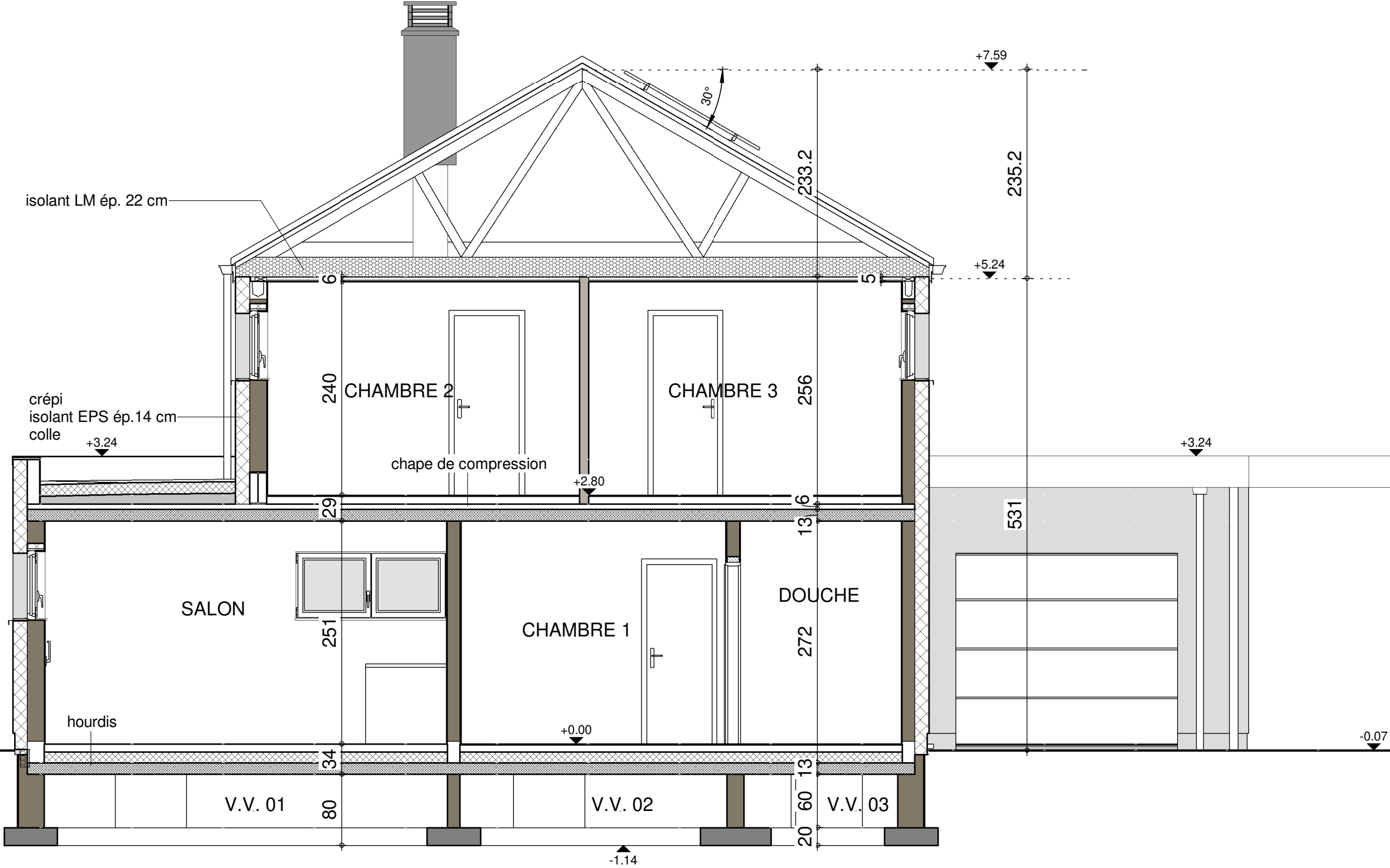
COUPE AA
